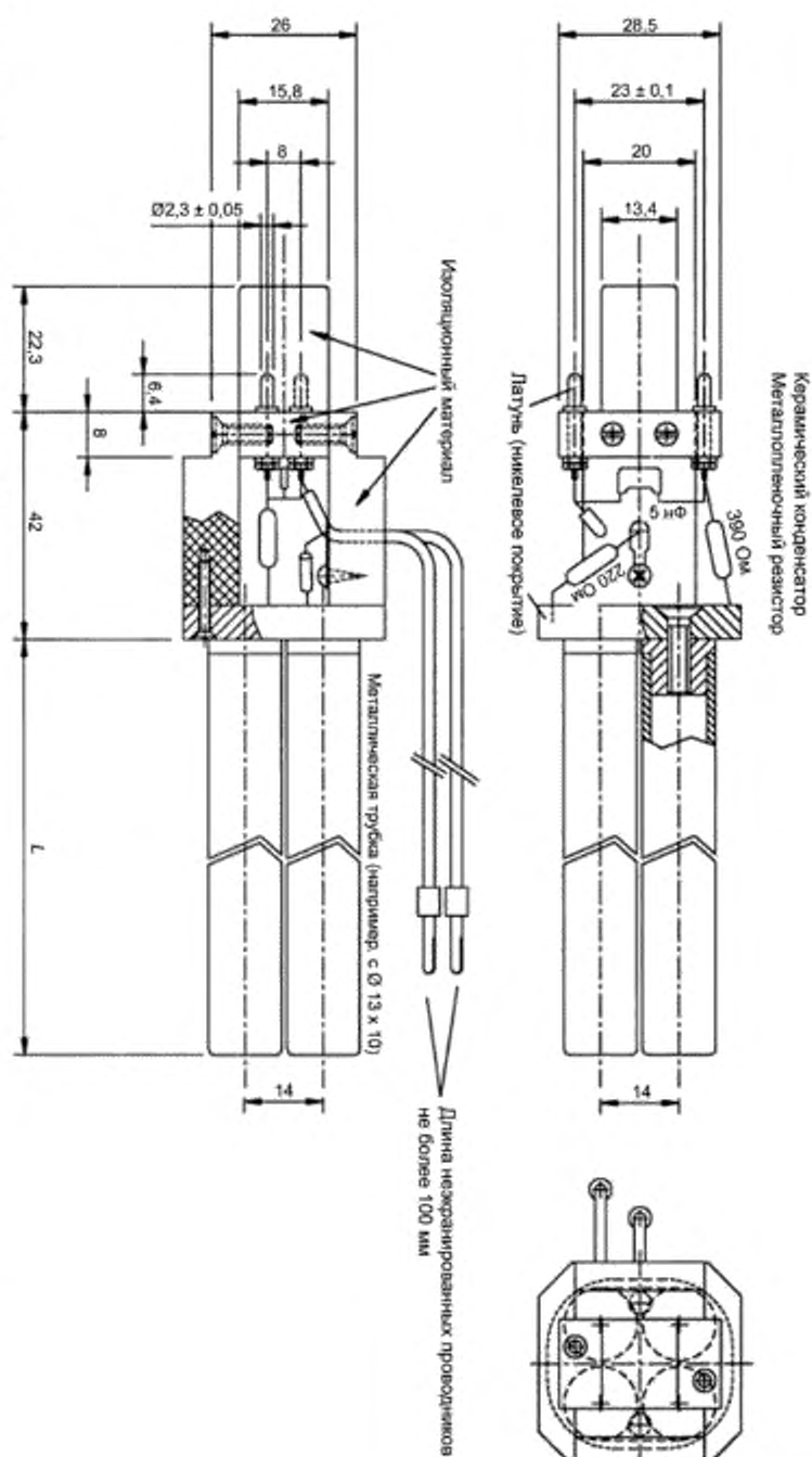
Рисунок 4f – Эквивалент однополюсной четырехпроводной линейной люминесцентной лампы с диаметром трубок 12 мм
