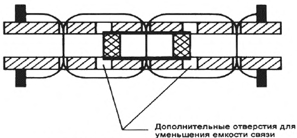
Рисунок A.2b – Детали конструкции сердечника трансформатора
