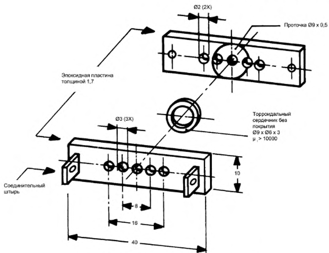
Рисунок A.2b – Детали конструкции сердечника трансформатора
