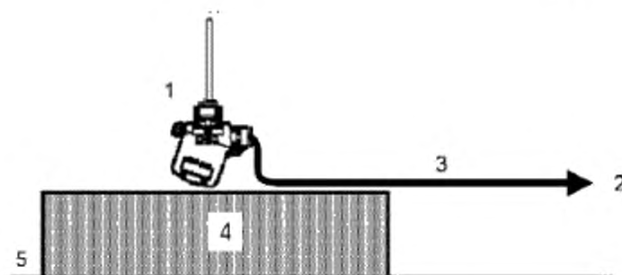
1 — датчик температуры (ориентация датчика приведена только в качестве примера); 2 — вспомогательное оборудование (например, блок питания, блок оценки сигнала или система передачи сигнала); 3 — соединительный кабель, неэкранированный, нескрученный, если не указано иное; 4 — изолирующая прокладка (размер согласно соответствующему основополагающему стандарту); 5 — эталонное заземление
