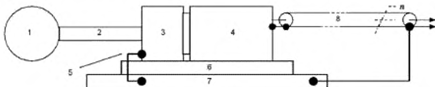
1 — рабочая среда; 2 — трубка; 3 — адаптер давления; 4 — датчик давления; 5 — заземление; 6 — изолирующая прокладка; 7 — эталонная земля; 8 — соединительные n линий
