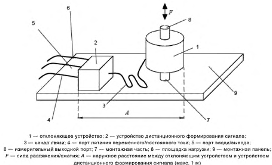
Рисунок АА.1 — Пример конфигурации датчика силы с дистанционным формированием сигнала
