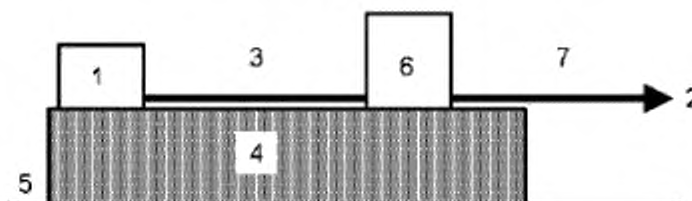
1 — датчик температуры; 2 — вспомогательное оборудование (например, блок питания, блок оценки сигнала); 3 — соединительный кабель, неэкранированный, нескрученный, если не указано иное; 4 — изолирующая прокладка (размер согласно соответствующему основополагающему стандарту); 5 — эталонное заземление; 6 — модуль формирования сигнала преобразователя; 7 — соединительный кабель, неэкранированный, нескрученный, если не указано иное
