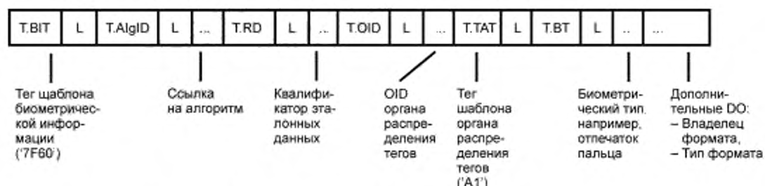
Рисунок В.5 — Пример шаблона биометрической информации (BIT)
