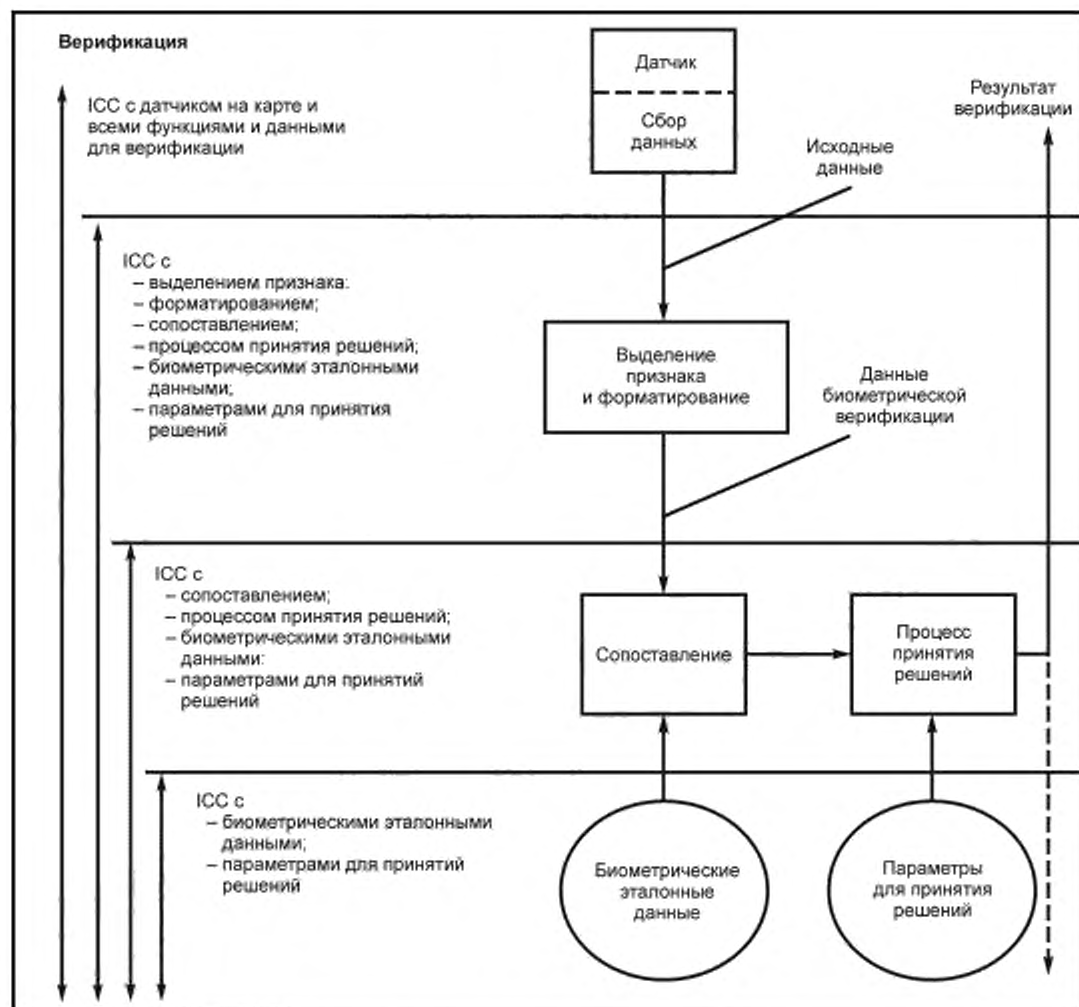
Рисунок А.2 — Общая схема процесса верификации
