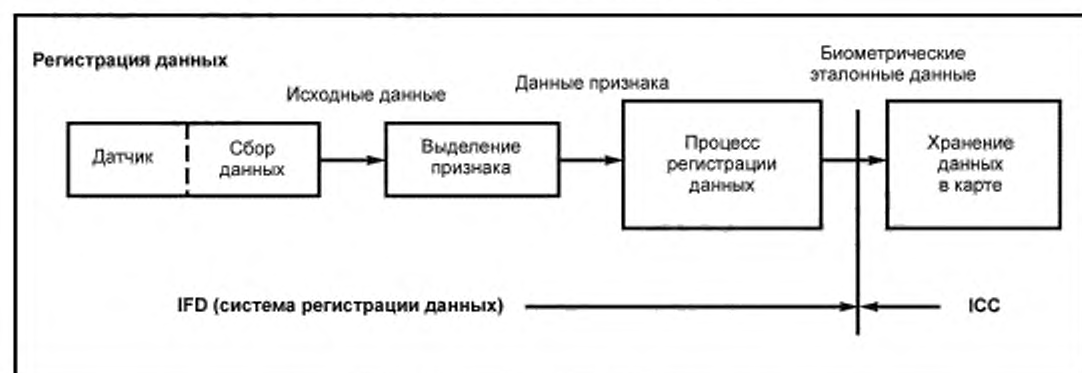
Рисунок A.1 — Общая схема процесса регистрации данных
