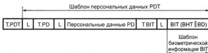
Рисунок D.3 — Шаблон персональных данных с BIT (пример)
