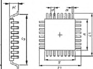
Рисунок 2, лист 4
