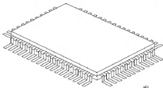
Рисунок 5 – Конструкция корпуса типа PQFP (прямоугольный)
