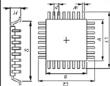
Рисунок 2, лист 2
