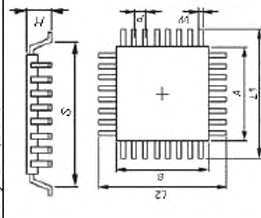
Рисунок 2, лист 3
