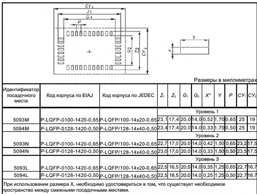
Рисунок 16 — Размеры посадочного места корпуса типа PLQFP (прямоугольный)
