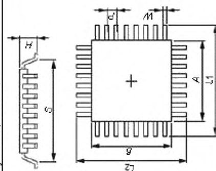
Рисунок 18, лист 2
