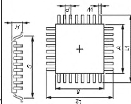
Рисунок 18, лист 3
