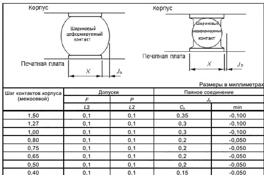
Рисунок 6 – Анализ формы паяного соединения
