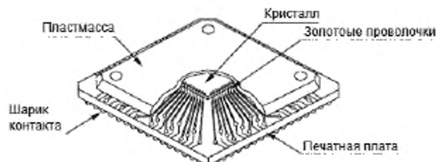
Рисунок 4 – Корпус BGA (квадратный)
