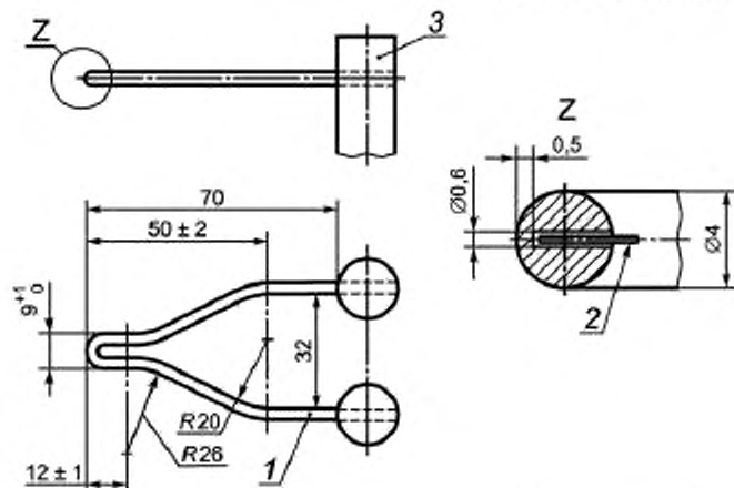
Рисунок 1 — Раскаленная проволока
