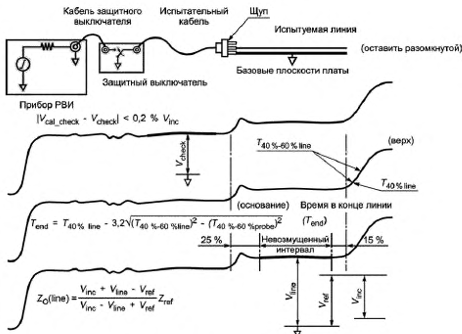
Рисунок 19 — Неискаженный интервал
