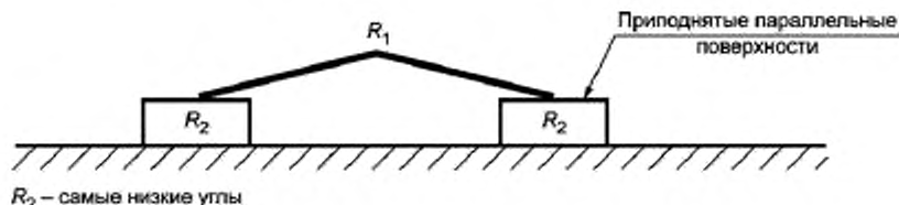
а) Схема измерения скручивания при арбитражном испытании, приподнятые параллельные поверхности
