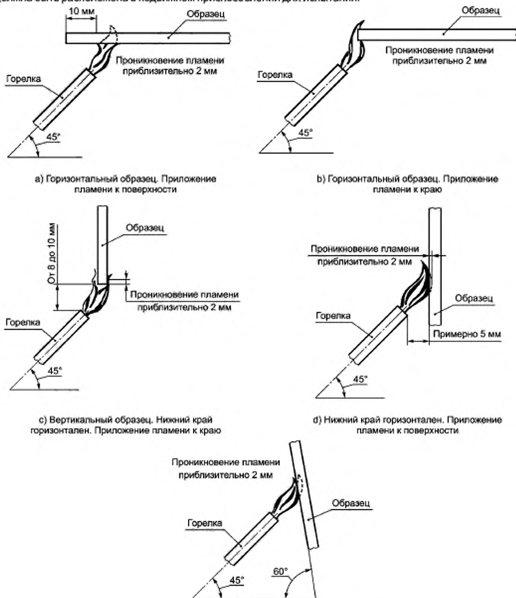
Рисунок 3 — Испытание с использованием горелки игольчатого типа
