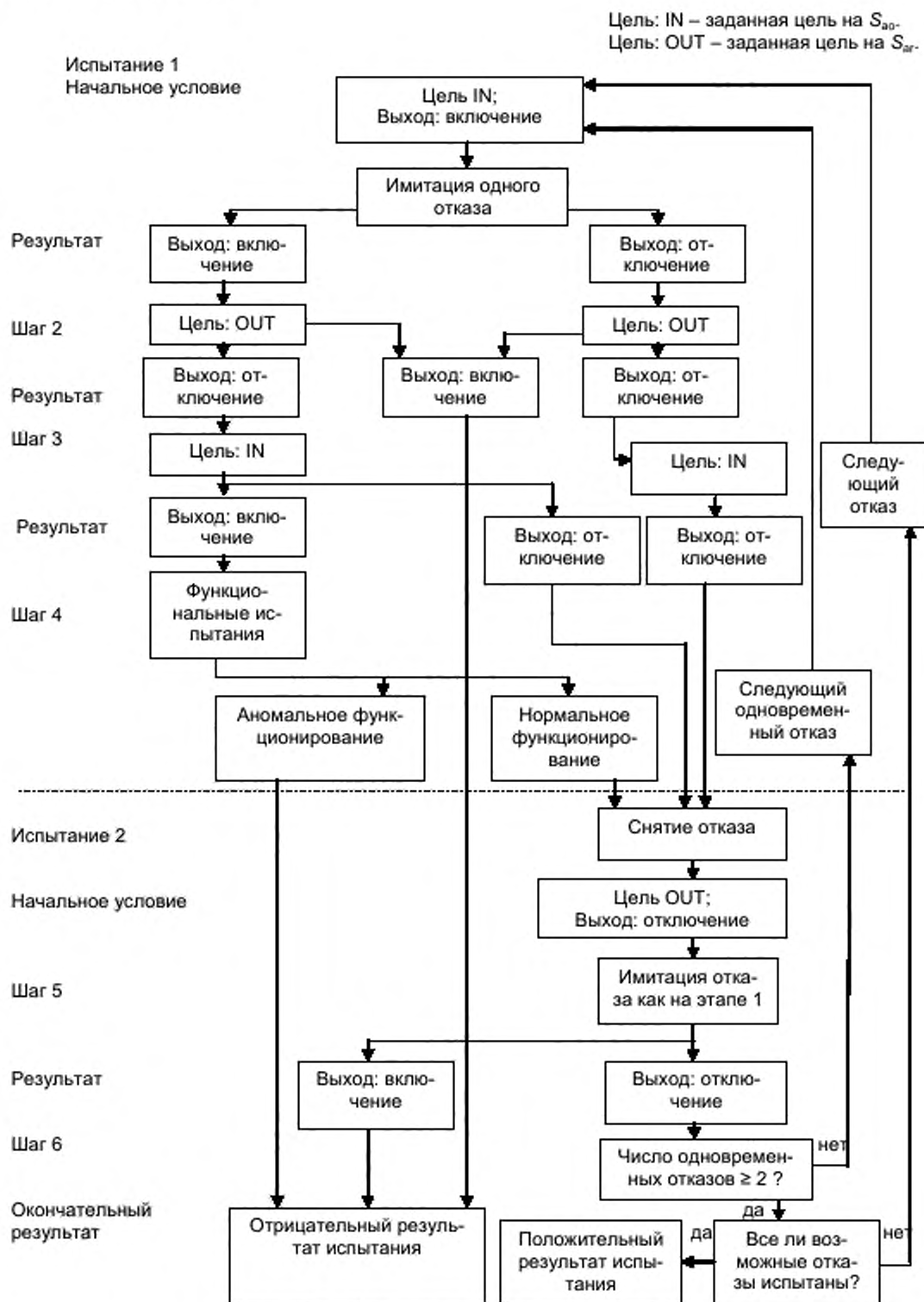
Рисунок А.3 – Последовательность испытаний для ОБД-М
