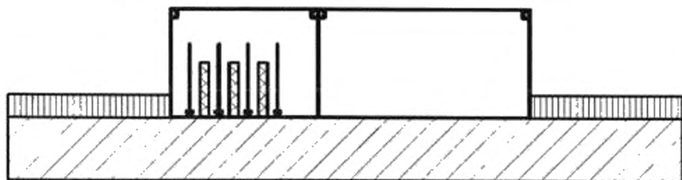
Рисунок АА.2 – Пример напольной установки шинопровода
