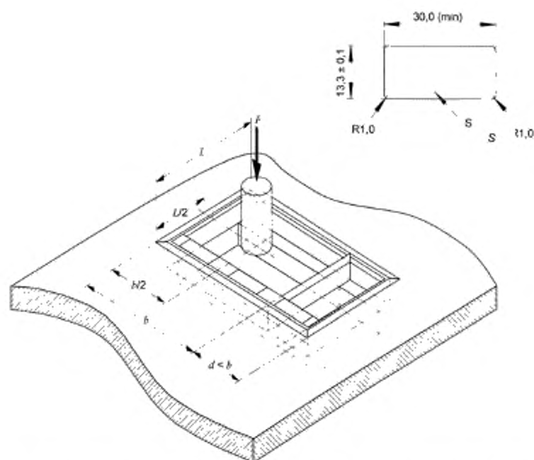
b – ширина наибольшего отсека; d – ширина наименьшего отсека; L – длина сервисного блока, установленного заподлицо с полом; F – вертикальное усилие, приложенное к цилиндру; S – размеры стального испытательного цилиндра
