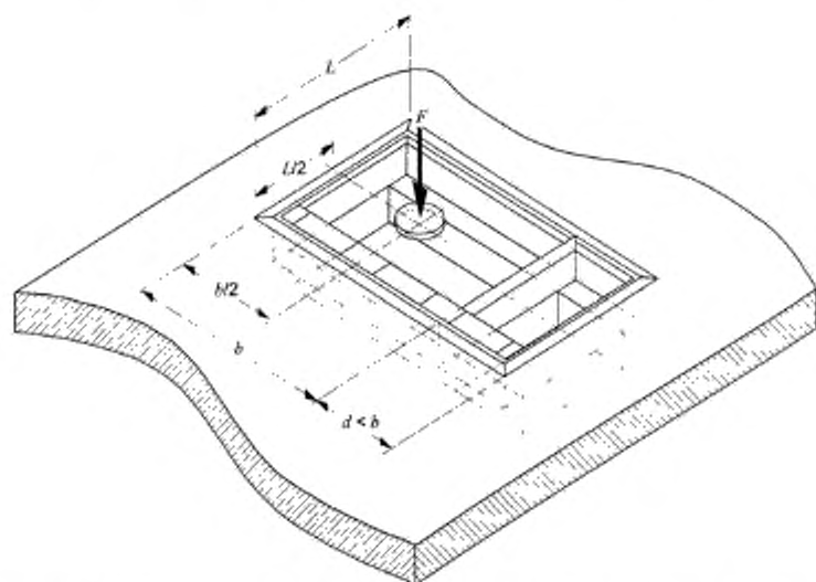
b – ширина наибольшего отсека; d – ширина наименьшего отсека; L – длина сервисного блока, установленного заподлицо с полом; F – вертикальное усилие, приложенное к цилиндру
