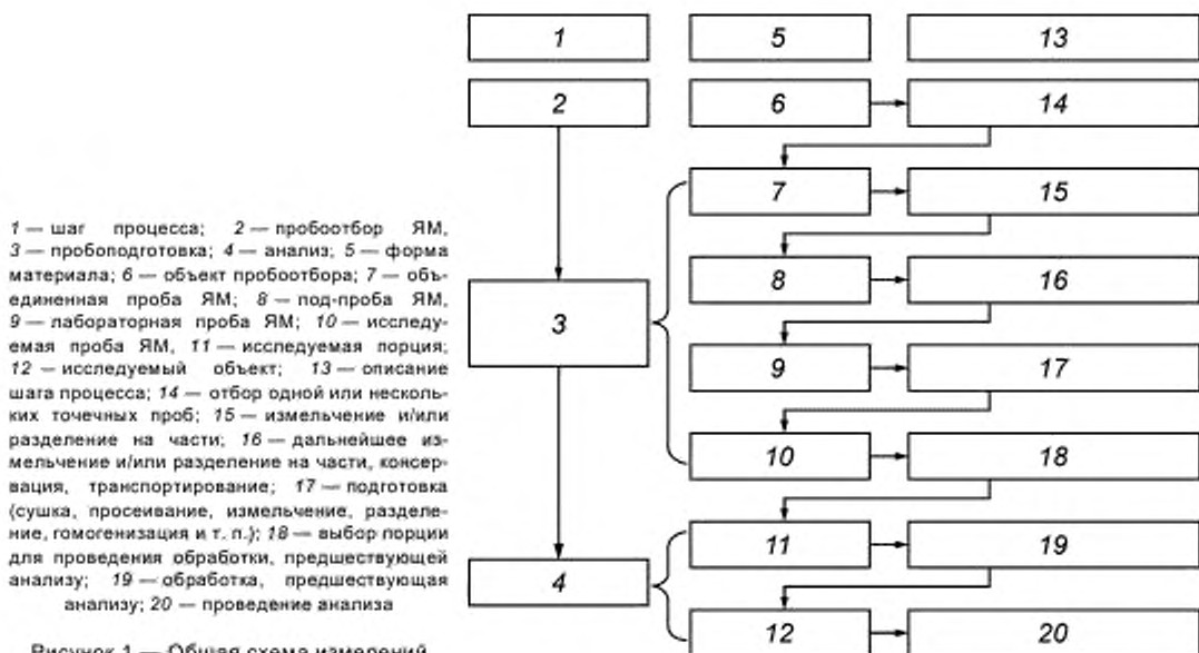
Рисунок 1 — Общая схема измерений
