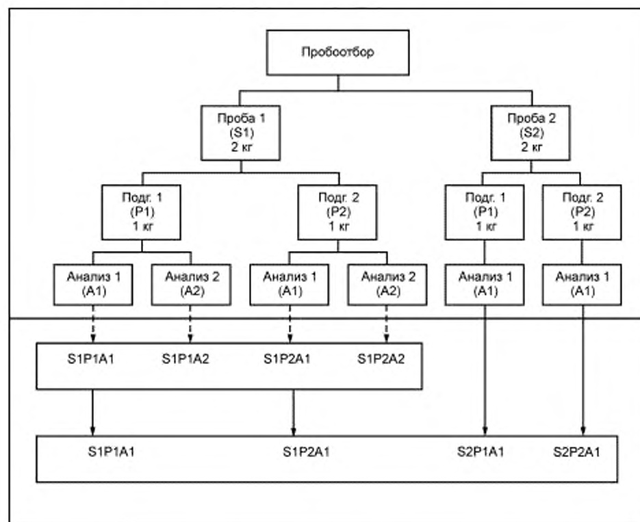
Рисунок А.1 — Альтернативный несбалансированный план
