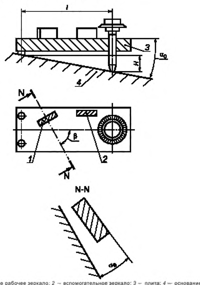
1 — плоское рабочее зеркало; 2 — вспомогательное зеркало; 3 — плита; 4 — основание
