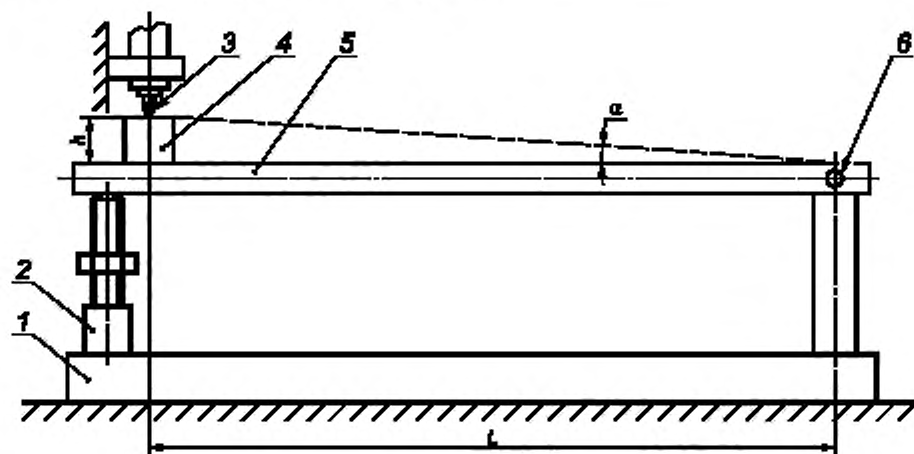
Рисунок В.1 — Схема экзаменатора
