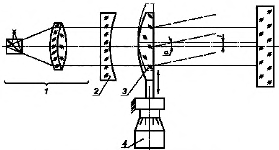
1 — автоколлиматор; 2, 3 — линзы ОЛК; 4 — микрометрический винт ОЛК
