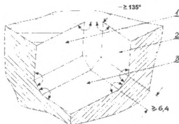
1, 2 и 3 – соединяемые поверхности
