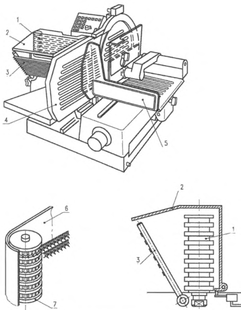
1 – разгрузочный транспортер; 2 – защитное ограждение с блокирующим устройством; 3 – укладчик; 4 – защитная пластина; 5 – держатель продукта; 6 – защитное ограждение возвратно-поступательного механизма; 7 – защитные диски
