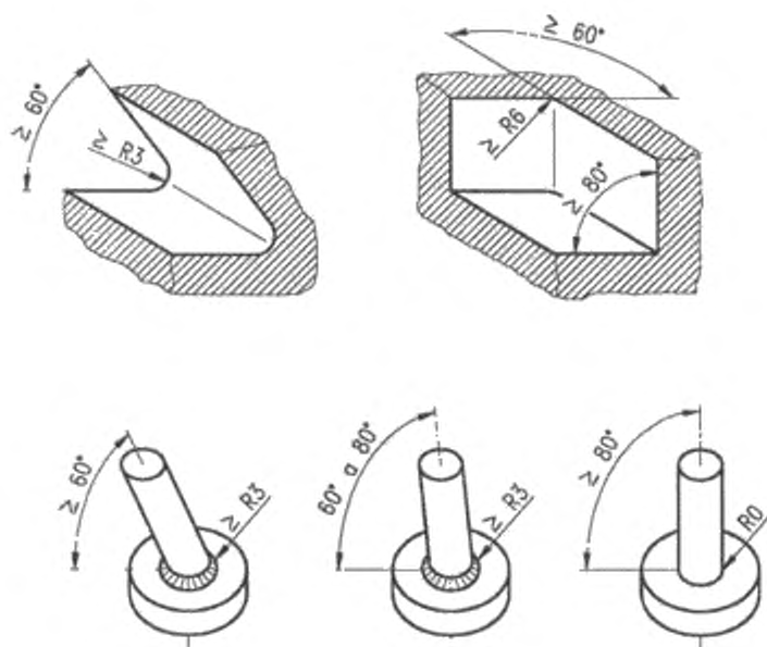
Рисунок 16 – Соединения в зоне разбрызгивания
