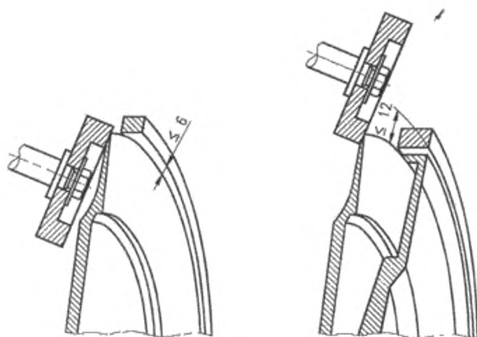
Рисунок 8b – Максимальные зазоры, при которых допускается заточка ножа
