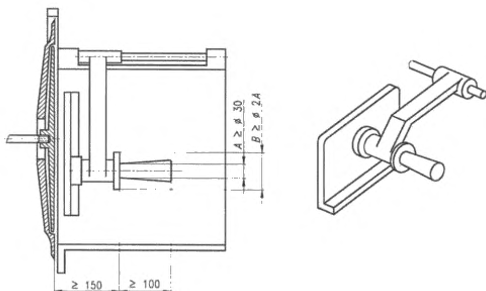
Рисунок 10 – Рукоятка толкателя
