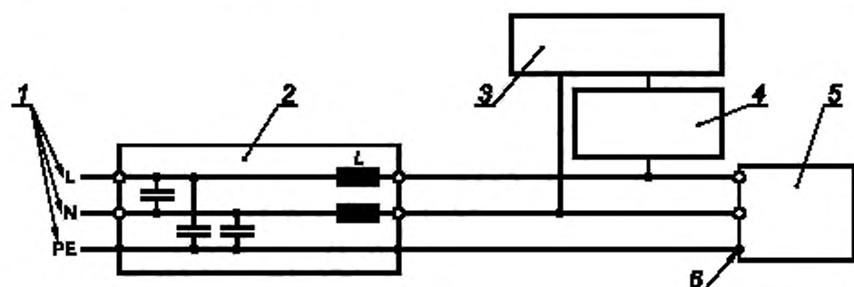
Рисунок 2 — Пример развязывающего фильтра для однофазной сети
