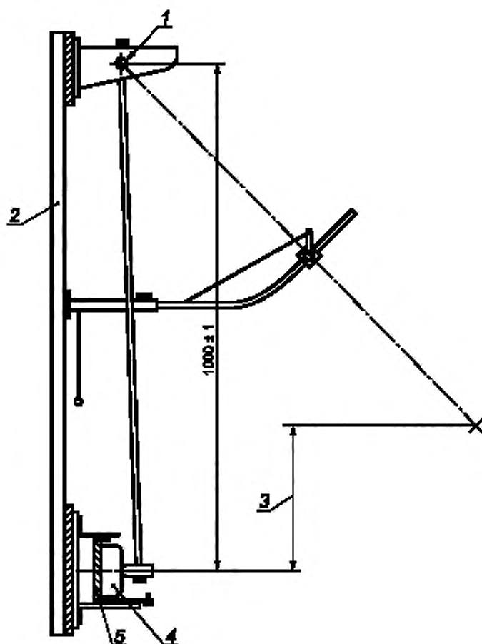
1 — маятник, 2 — рама; 3 — высота падения; 4 — образец, 5 — монтажный крепеж
