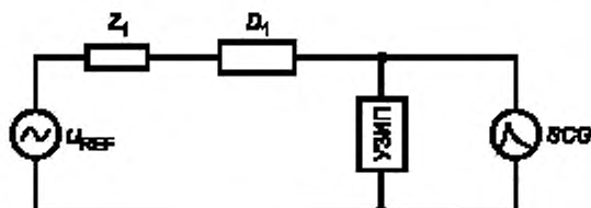
Z_1 — полное сопротивление для регулирования ожидаемого тока короткого замыкания согласно таблице 8; D_1 — внешний разъединитель УЗИП; SCG — генератор импульсов тока с развязывающим фильтром
