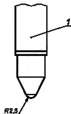
1 — нагрузочный стержень
