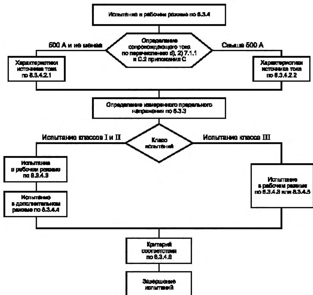
Рисунок 6 — Схема испытания в рабочем режиме
