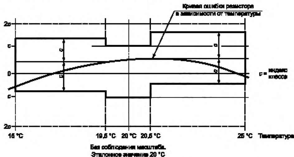
Рисунок 1 — Влияние температуры
