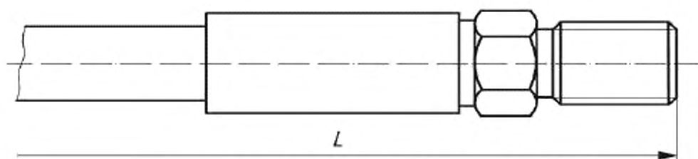
Рисунок 9 — Длина до ниппеля для присоединения рукава
