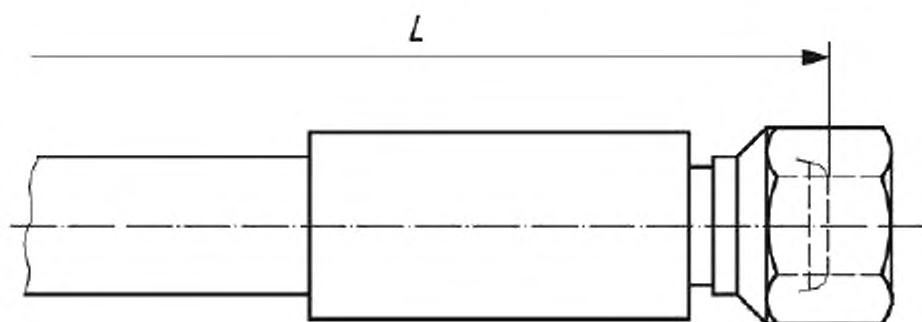
Рисунок 5 — Длина рукава между обжимными муфтами
