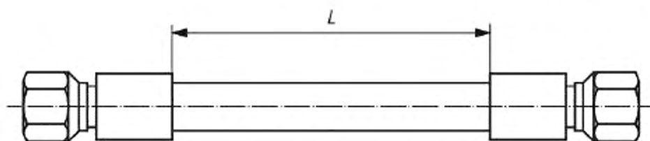
Рисунок 5 — Длина рукава между обжимными муфтами
