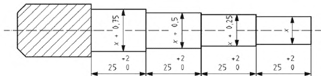
Рисунок 1 — Калибры-пробки
