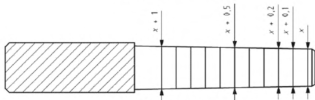
Рисунок 2 — Конусные калибры
