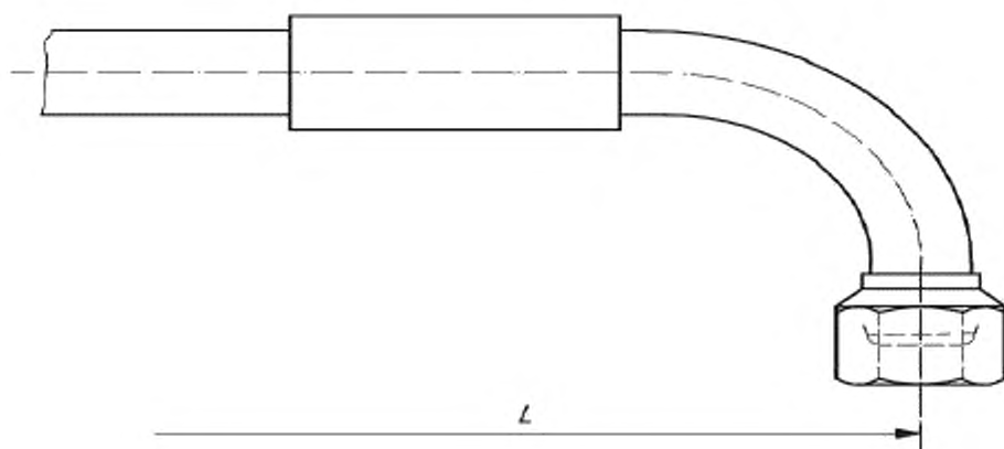
Рисунок 6 — Длина до nipples для присоединения рукава
