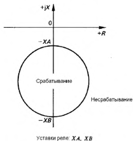
Рисунок 1f — Круговая смещенная характеристика
