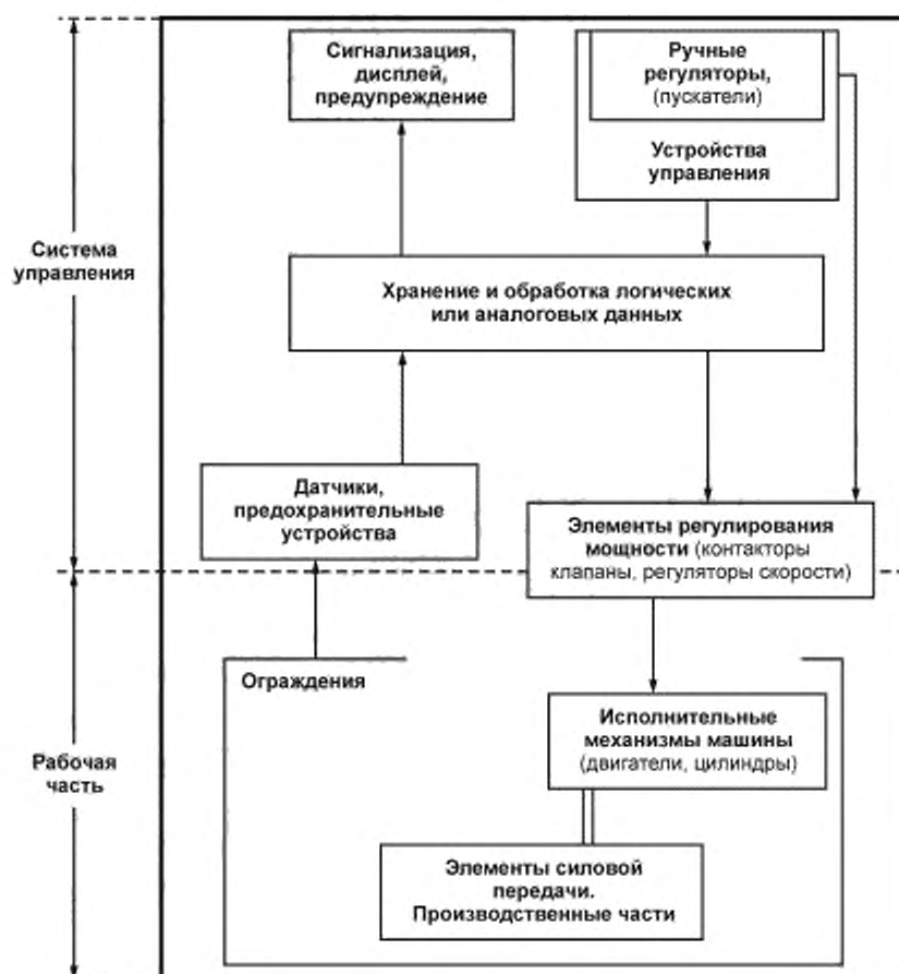
Рисунок А.1 — Общее схематическое изображение машины
