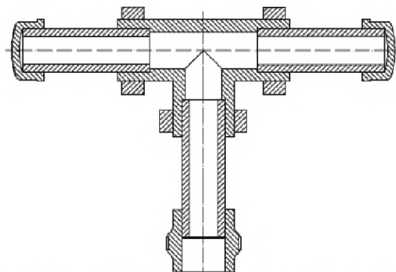
Рисунок 1 – Пример герметизации испытываемого образца с осевой нагрузкой, возникающей под действием гидростатического давления
