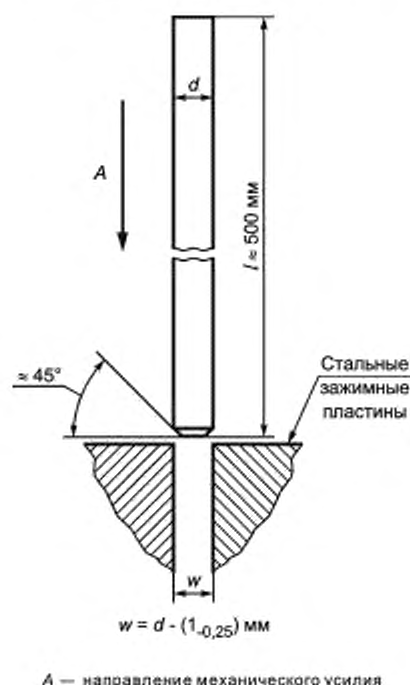
Рисунок 2 — Пример испытания адгезии
