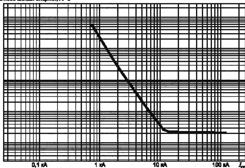
Отпущенная энергия, А 2 ·с
