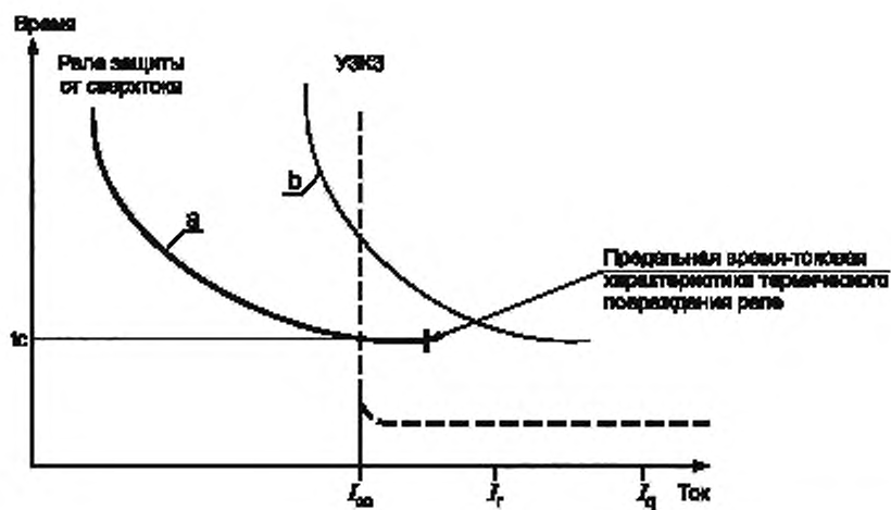
Рисунок 5b — Координация пускателя с автоматическим выключателем
