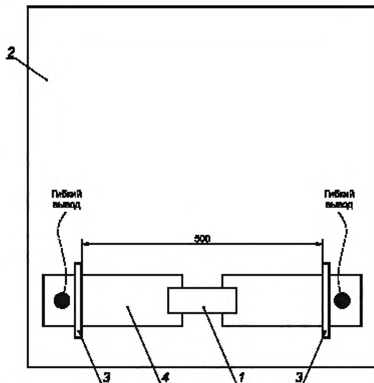
Рисунок 3 — Пример соединения перемычкой
