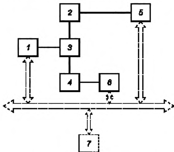
1 — источник напряжения постоянного/переменного тока; 2 — эталонный ПН; 3 — тройниковый соединительный элемент; 4 — поверяемый ПН; 5, 6 — вольтметр постоянного тока; 7 — ПЭВМ
