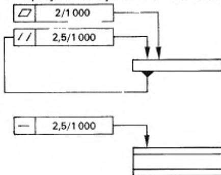
Рисунок A.8 – Допуски на форму
