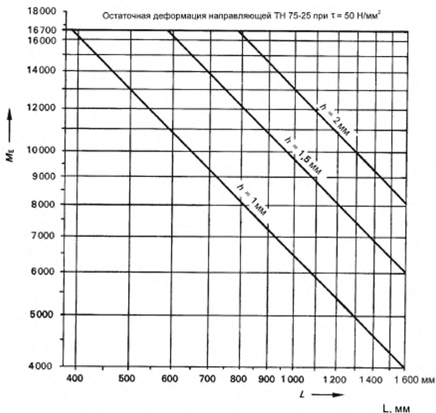
Рисунок В.3 – Допустимая нагрузка m_c = f(L, h)
