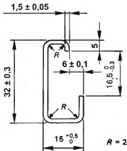
Рисунок A.9 – Размеры направляющих G-образного профиля
