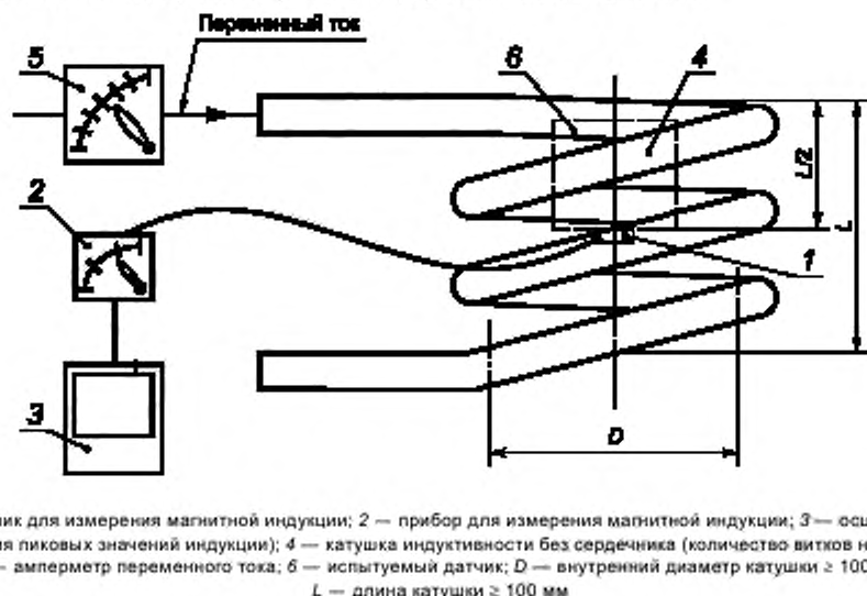
Рисунок Е.1 — Примерная испытательная схема для проверки устойчивости датчика к воздействию переменного магнитного поля
