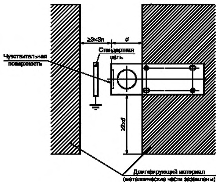
Рисунок A.2 (CC) — Установка (монтаж)
