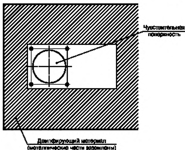
Рисунок A.2 (CD) — Установка (монтаж)
