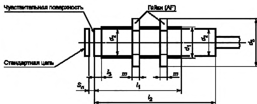
Рисунок А.1 (IА) — Габаритные размеры
