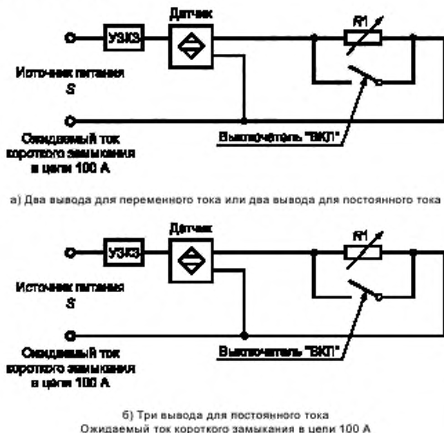
Рисунок 10 — Схема испытаний на короткое замыкание (8.3.4.2)
