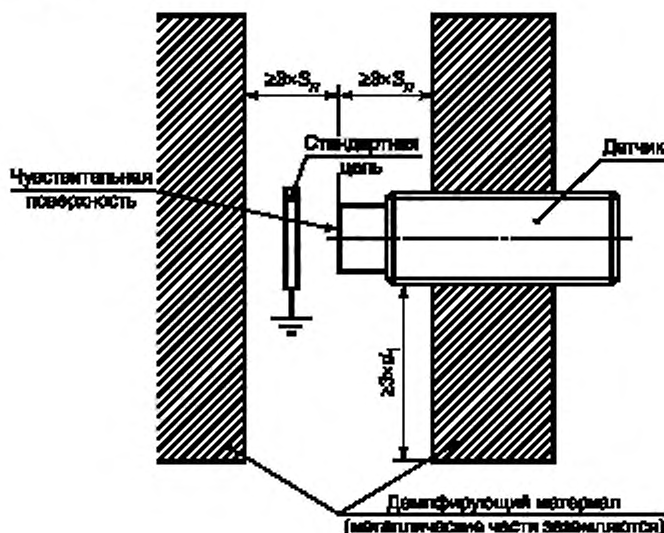
Рисунок A.2 (CA) — Установка (монтаж)
