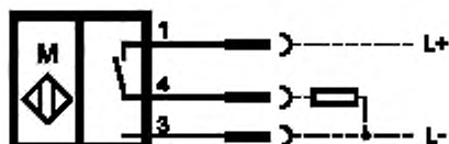
Рисунок F.1 — Примеры символов бесконтактных датчиков
