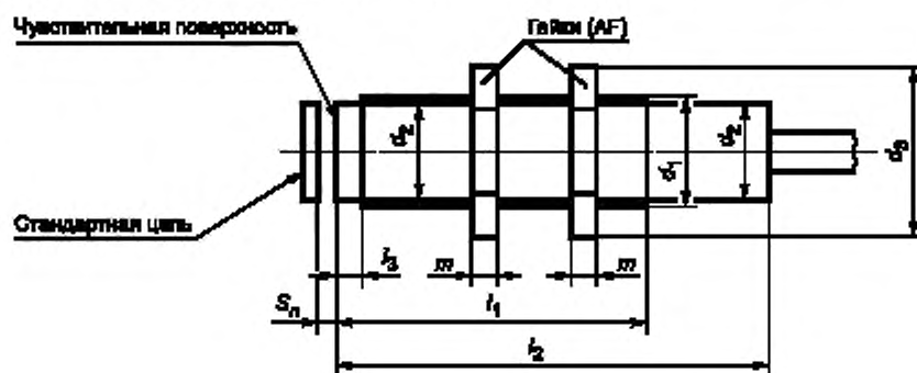
Рисунок А.1 (СА) — Габаритные размеры
