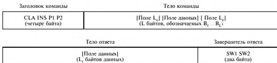
Рисунок 8 — Структуры APDU-сообщений
