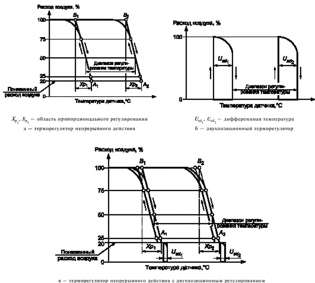
Рисунок 2 — Типовые характеристики терморегуляторов
