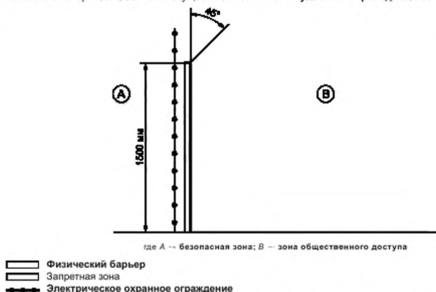
Рисунок СС.1 — Запретная зона для импульсных проводников
