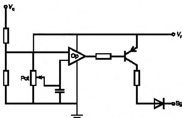
где V_c — напряжение зарядки; V_r — сравниваемое напряжение; Sg — стробирующий импульс; Pot — регулятор переключения скорости; Op — компаратор
