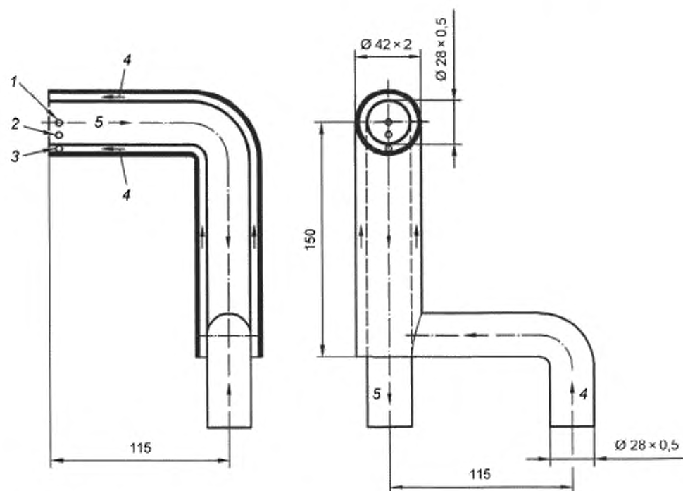
Рисунок 6 — Типичная схема альтернативного соединения для головы-манекена
