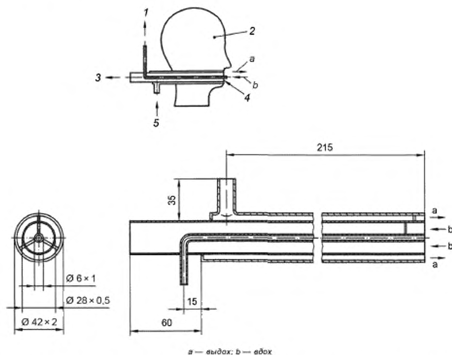
Рисунок 5 — Голова Шеффилда — макет, предназначенный для определения содержания диоксида углерода во вдыхаемом воздухе, с трубкой для измерения сопротивления дыханию
