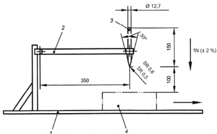
Рисунок 1 — Схема типового оборудования для испытаний на стойкость к проколам и разрывам
