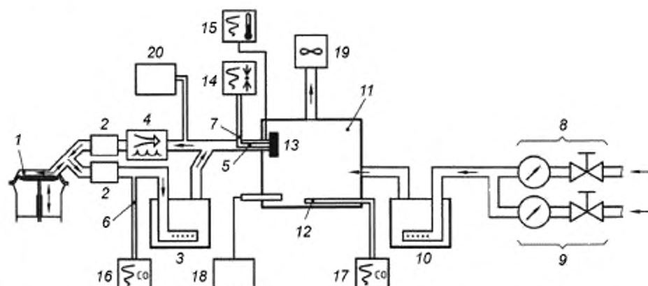
1 — дыхательная машина; 2 — электромагнитные клапаны; 3 — увлажнитель (выдыхаемый воздух); 4 — холодильник; 5 — адаптер; 6 — пробоотборник для взятия проб на монооксид углерода (выдыхаемый воздух); 7 — диафрагма датчика давления; 8 — измеритель потока испытательной атмосферы; 9 — измеритель потока монооксида углерода; 10 — увлажнитель (испытательная атмосфера); 11 — испытательная камера (приблизительные размеры 30 × 30 × 26 см); 12 — пробоотборник для определения содержания монооксида углерода в испытательной атмосфере на входе фильтрующего самоспасателя; 13 — испытуемый образец (максимальная разность давлений на входе фильтрующего самоспасателя по отношению к давлению среды в испытательной камере 50 Па); 14 — датчик давления с регистратором; 15 — средство измерения температуры с регистратором; 16 — анализатор монооксида углерода и устройство записи (выдыхаемый воздух, см 3 /м 3 и см 3 ); 17 — анализатор монооксида углерода (испытательная атмосфера); 18 — измеритель влажности (испытательная атмосфера); 19 — сброс; 20 — измеритель влажности (выдыхаемый воздух)
