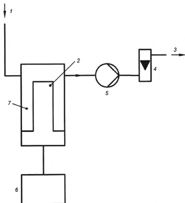
Рисунок А.1 — Схема для определения температуры вдыхаемого воздуха по влажному термометру
