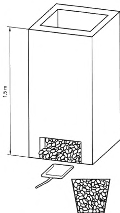
Рисунок 2 — Корзина и контейнер с резиновой стружкой
