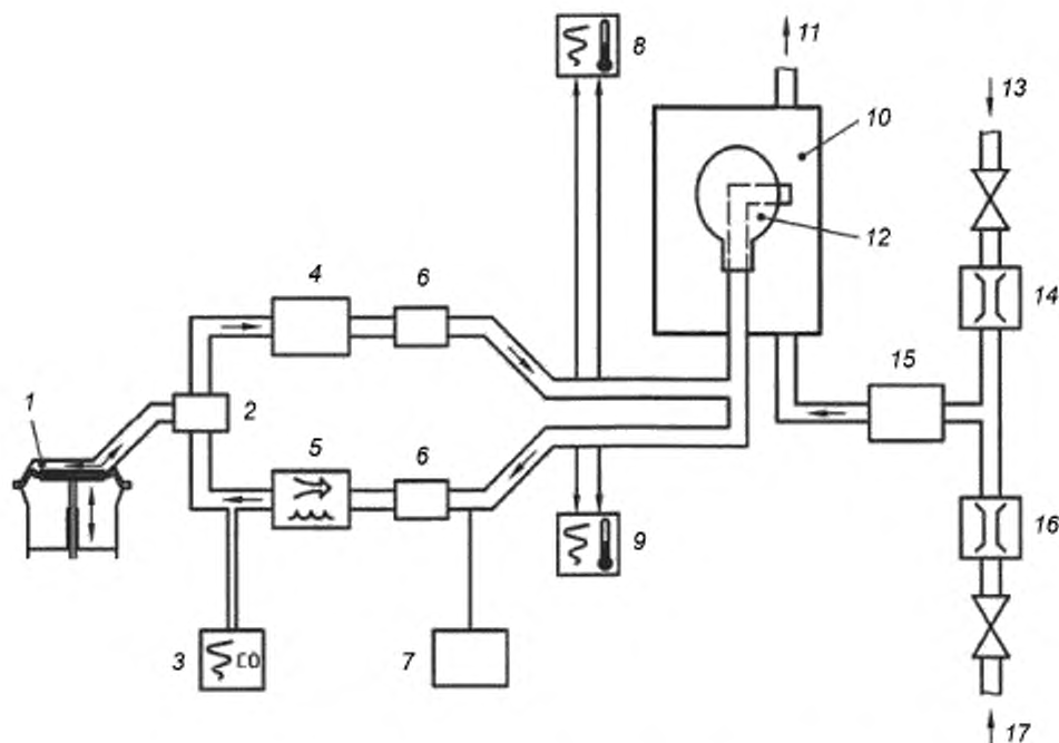
1 — дыхательная машина; 2 — система клапанов; 3 — анализатор монооксида углерода; 4 — увлажнитель; 5 — холодильник; 6 — электромагнитные клапаны; 7 — измеритель точки росы; 8 — средства измерения температуры и давления выдыхаемого воздуха; 9 — средства измерения температуры и давления вдыхаемого воздуха; 10 — испытательная камера; 11 — сброс, 12 — макет головы для фильтрующего самоспасателя; 13 — подача монооксида углерода; 14 — измеритель скорости потока; 15 — увлажнитель; 16 — измеритель скорости потока; 17 — сброс воздуха
