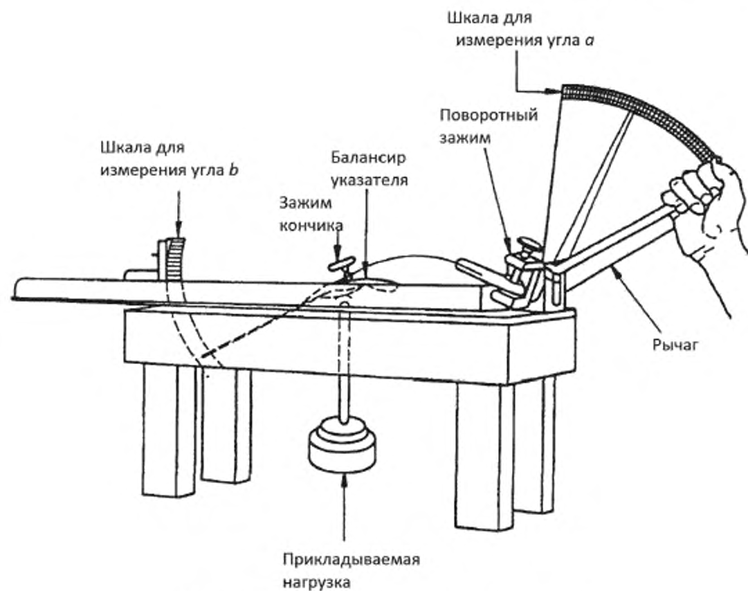
Рисунок А.2 — Установка для испытания ножей на прочность
