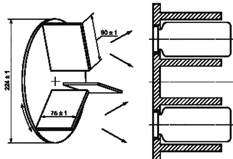
Рисунок 1 — Общая схема машины для испытания
