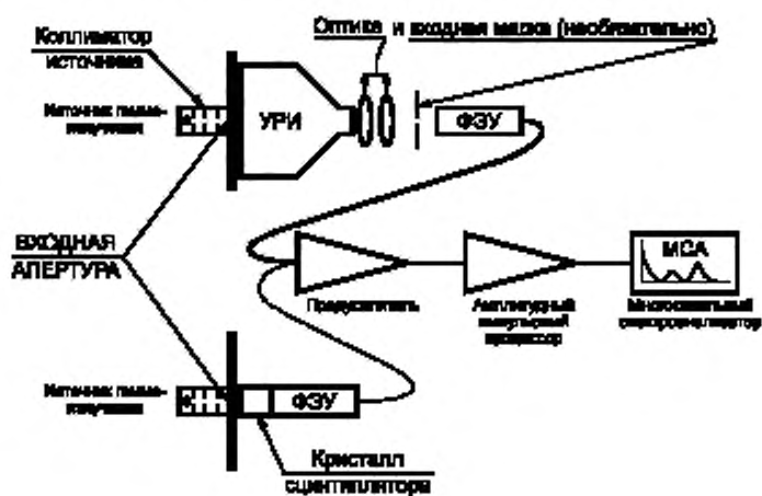
Типовая схема проведения испытаний
