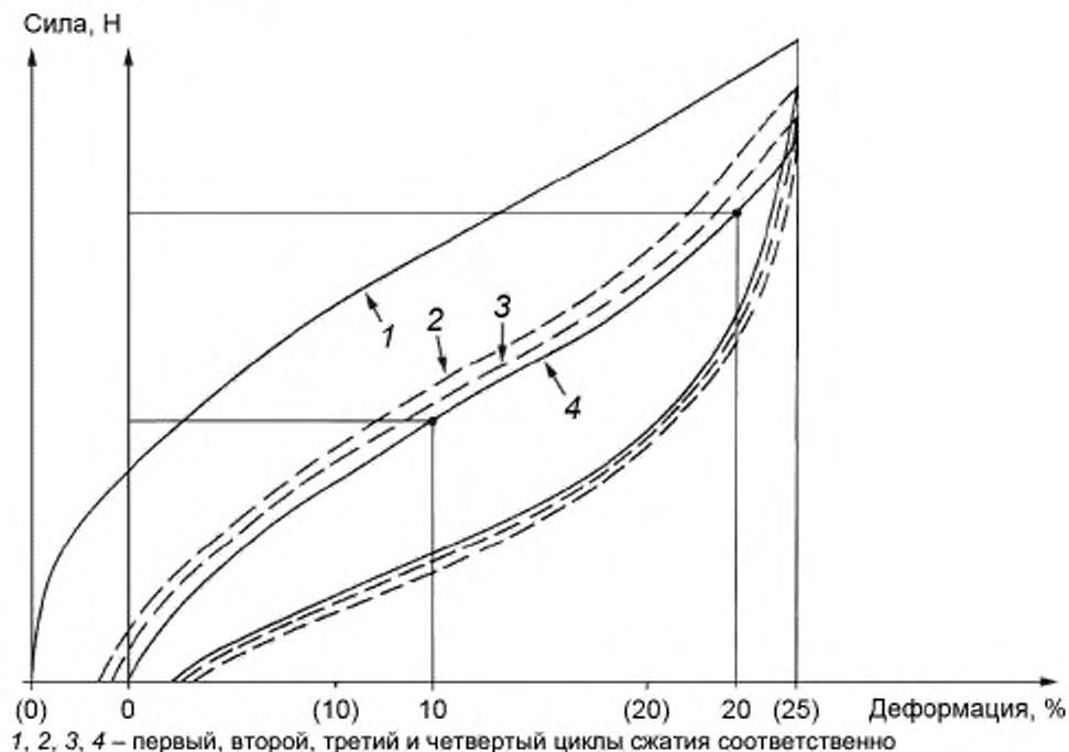
Рисунок 1 – Вычисление модуля сжатия
