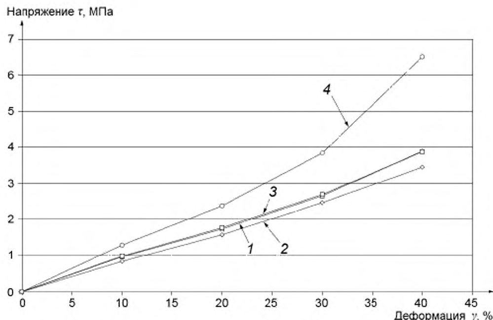
1, 2, 3, 4 – первый, второй, третий и четвертый образцы соответственно Рисунок А.2 – Статические упругопропрочностные свойства при сжатии приклеенных образцов для испытания (напряжения приведены без поправок)
