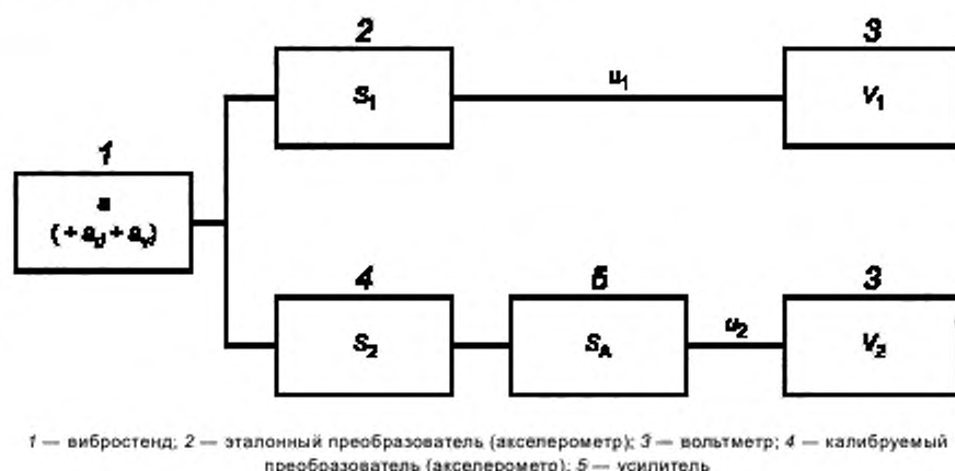
Рисунок D.1 — Схема процесса измерений
