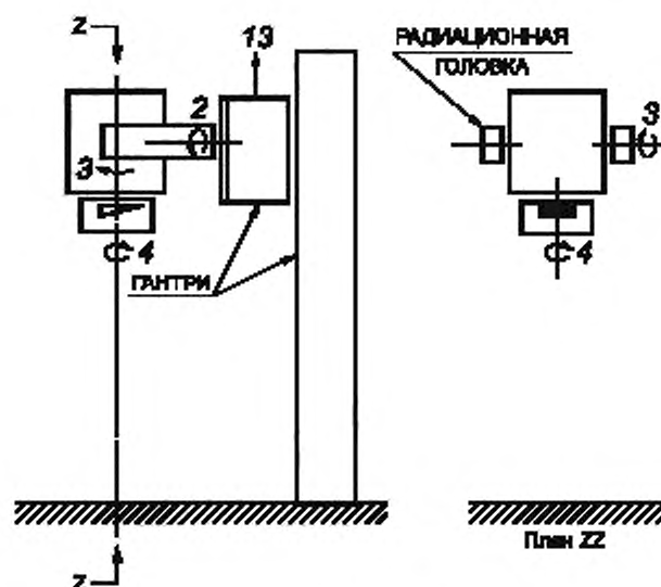
Рисунок 2 — Поворотный ГАНТРИ
