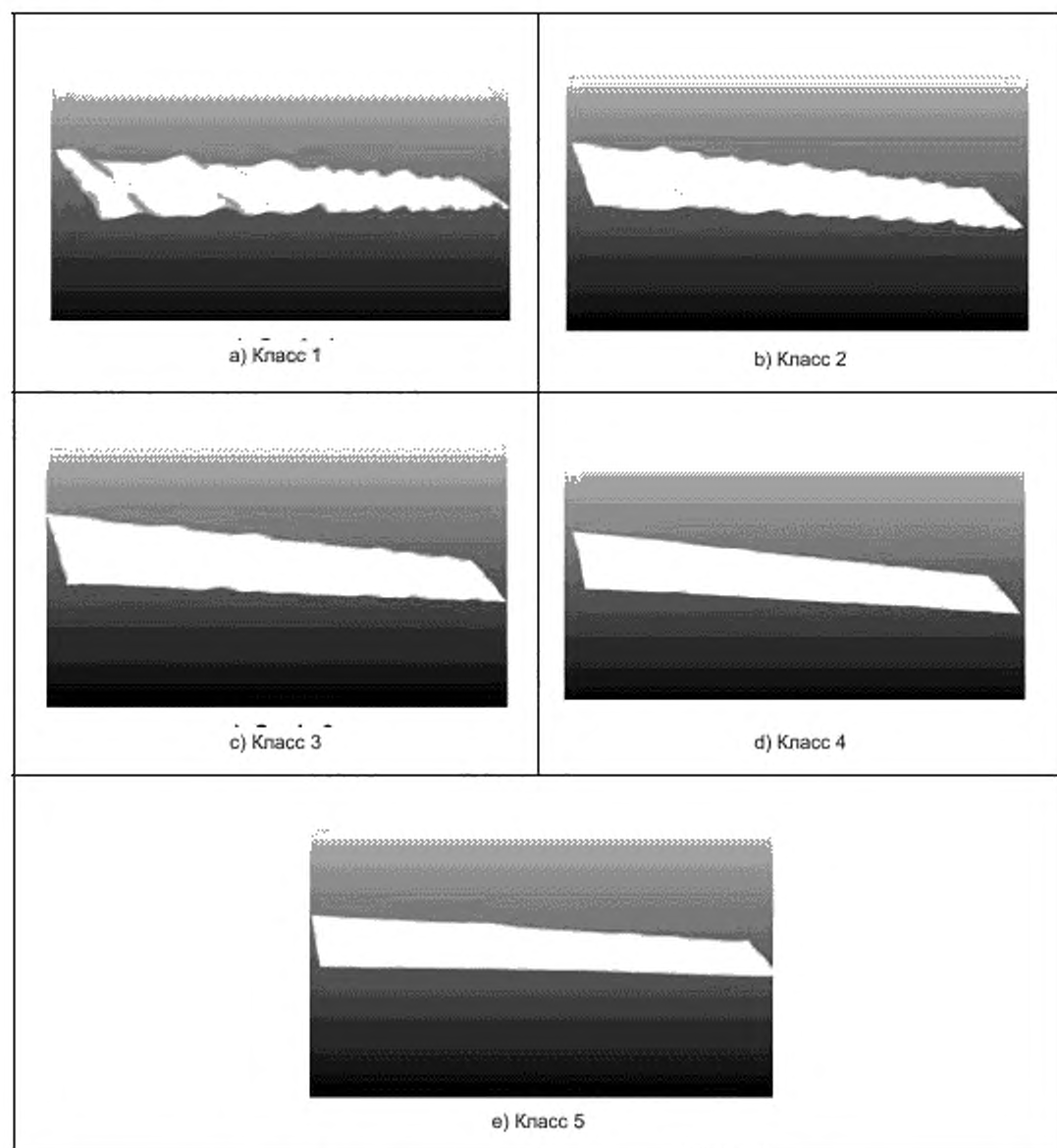
Рисунок А.10 — Измеренные изображения эталонов двойных швов
