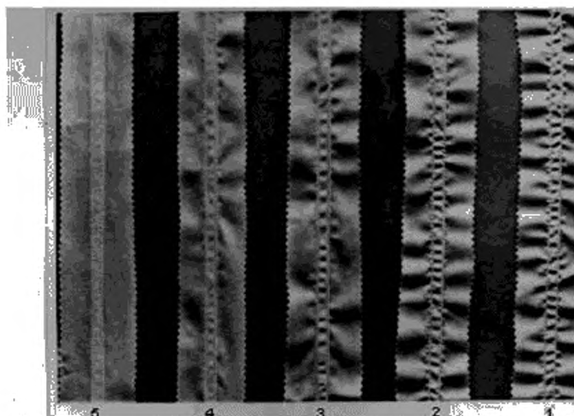
Рисунок 3 — Фотография сравнительной шкалы для двойных швов
