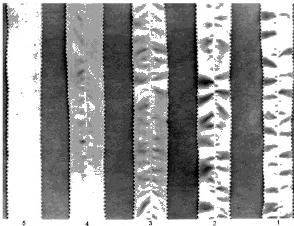
Рисунок 2 — Фотография сравнительной шкалы для одинарных швов
