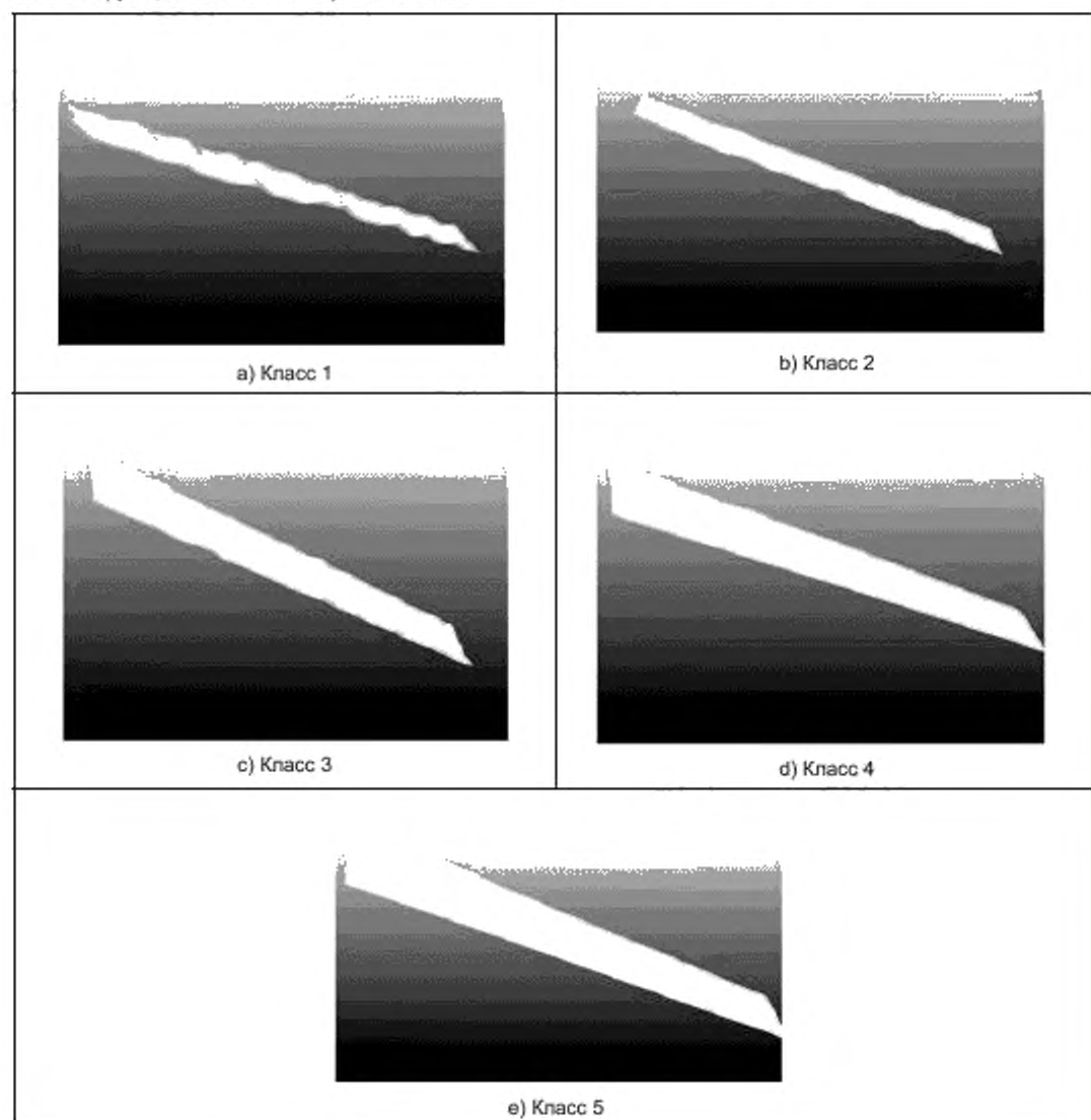
Рисунок А.3 — Измеренные изображения эталонов одинарных швов
