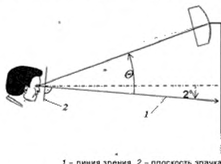
Рисунок А.1 – Угол между линией зрения наблюдателя и направлением падающего луча от индивидуального светильника
