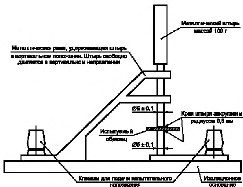
Рисунок 6 — Установка для испытаний на электрическую прочность
