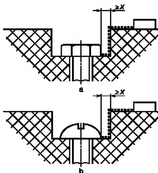
Рисунок Е.10 — Большое углубление
