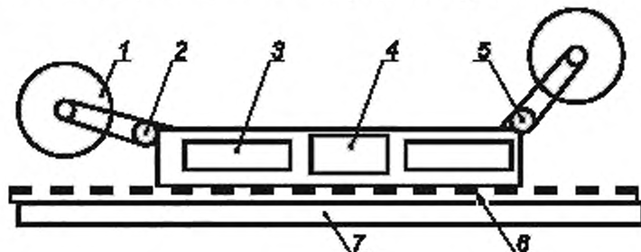
1 — шнек с резаками; 2 — поворотный редуктор; 3 — отделение редуктора; 4 — распределительное устройство; 5 — электродвигатель привода шнека; 6 — расположение реечной передачи; 7 — забойный скребковый конвейер
