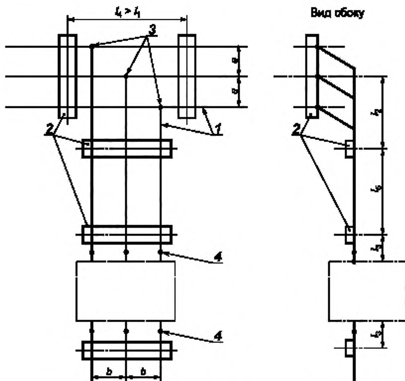
1 — шины; 2 — опоры; 3 — соединения шин; 4 — выводы подсоединения аппаратов; a, b, l_1, \dots, l_5 — размеры элементов конструкции
