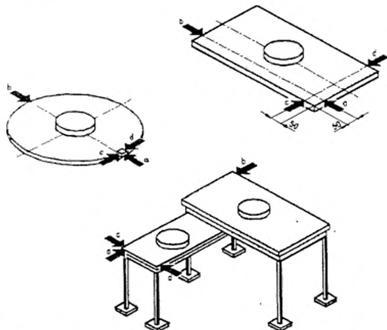
Рисунок 5 – Испытание на долговечность под действием горизонтальной нагрузки
