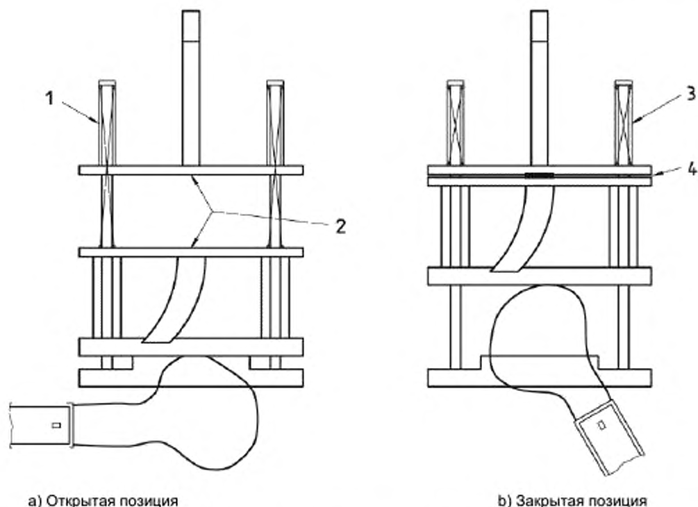
1 – натянутые пружины; 2 – открытый промежуток 0,5 см или 0,798 см в диаметре; 3 – сжатые пружины; 4 – испытуемая ткань
