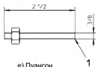
е) Пуансон
