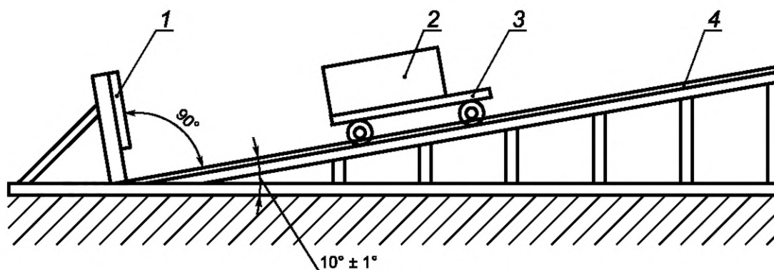
1 — ударная стенка (амортизирующий буфер); 2 — испытуемый образец; 3 — тележка; 4 — двухрельсовый стальной путь
