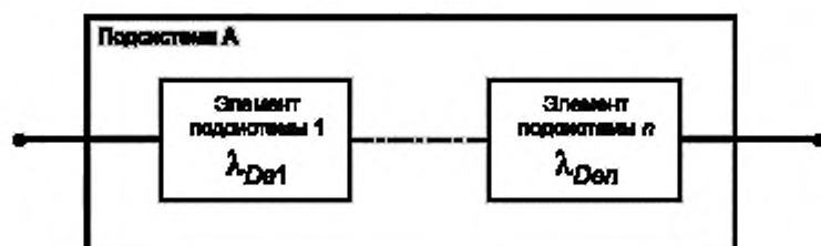
Рисунок 6 — Логическое представление подсистемы типа А
