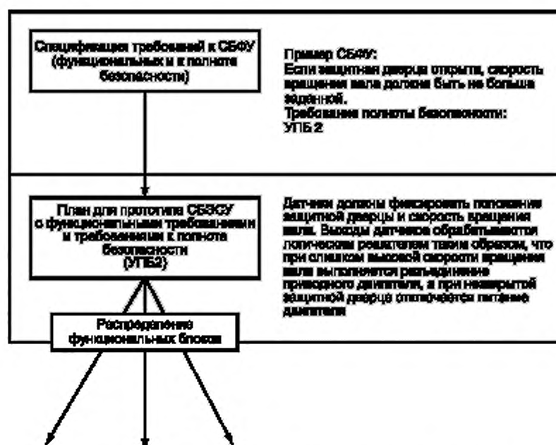
Рисунок В.4 — Декомпозиция в структуру функциональных блоков
