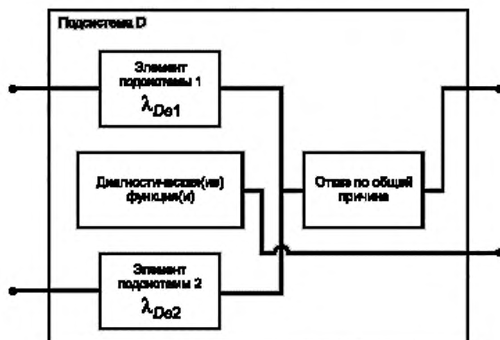
Рисунок 9 — Логическое представление подсистемы типа D
