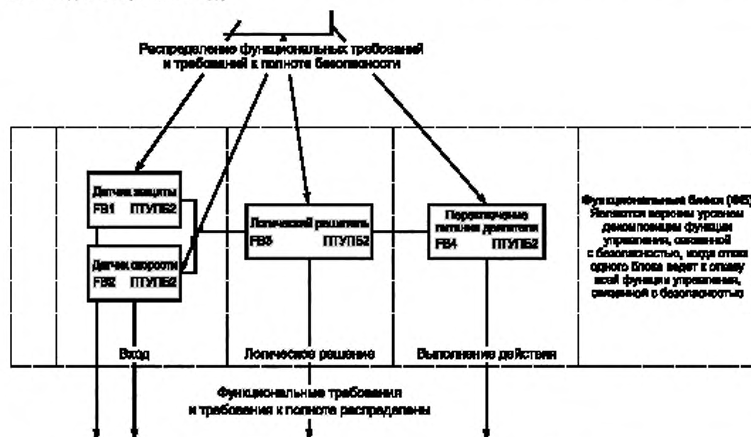
Рисунок В.5 — Начальная концепция архитектуры СБСУ
