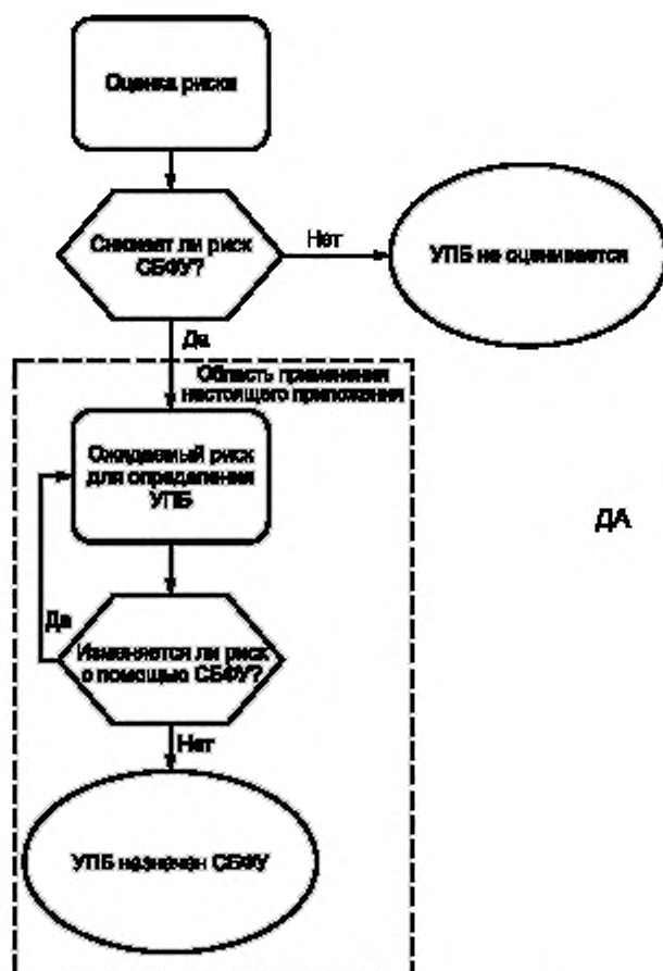
Рисунок А.1 — Структура процесса оценки УПБ
