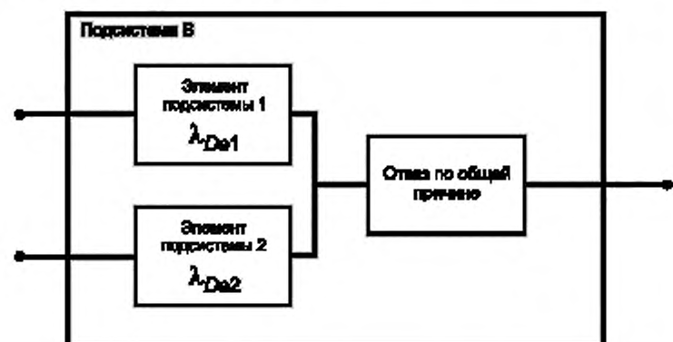
Рисунок 7 — Логическое представление подсистемы типа В
