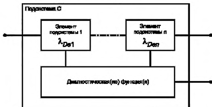
Рисунок 8 — Логическое представление подсистемы типа С
