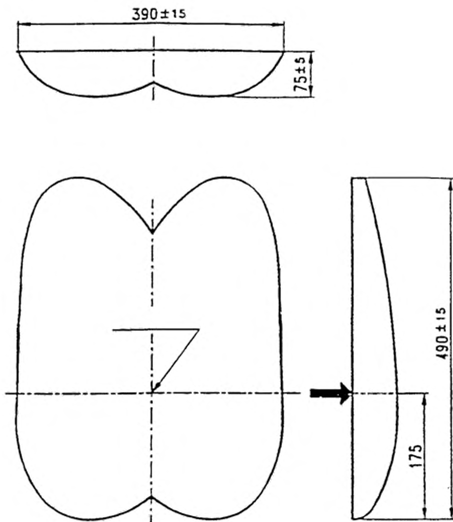
Рисунок 4 — Размеры нагрузочного штампа для сиденья
