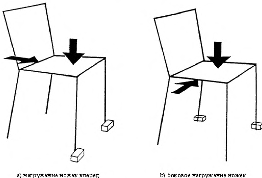
Рисунок 14 — Испытание ножек под действием статической нагрузки
