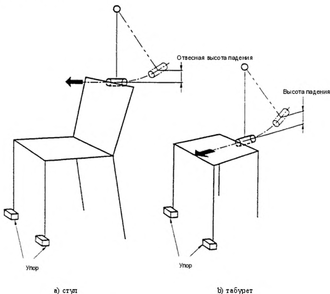
Рисунок 17 — Испытание спинки на удар
