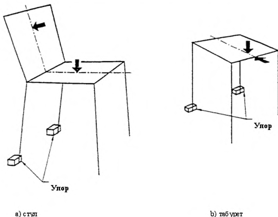
Рисунок 10 — Испытание сиденья и спинки под действием статической нагрузки
