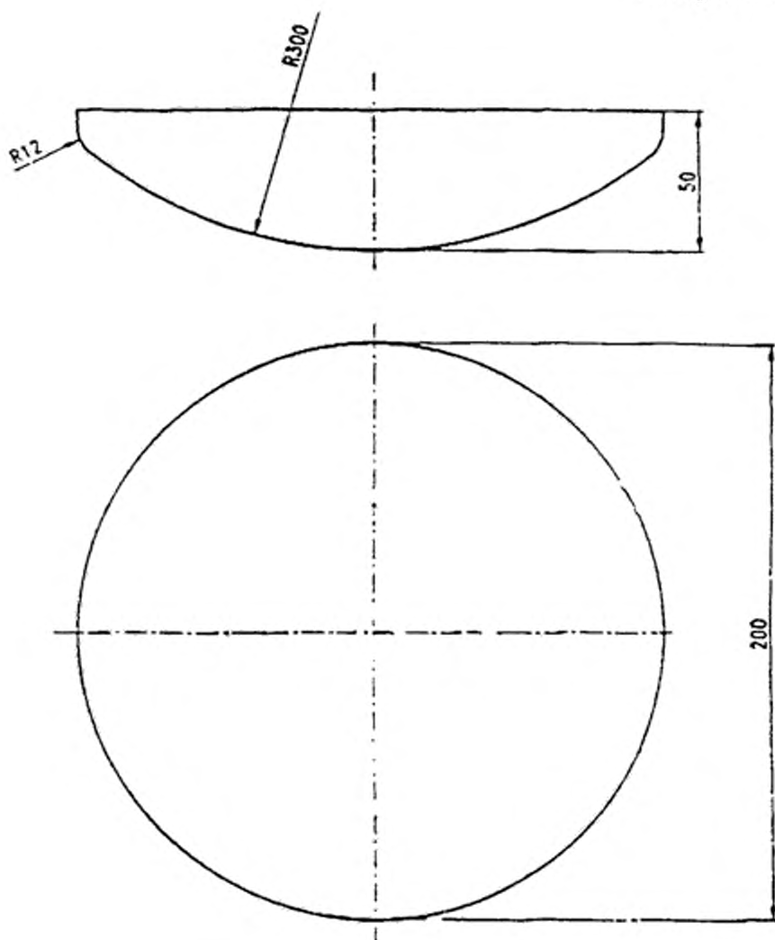
Рисунок 5 — Малый нагрузочный штамп
