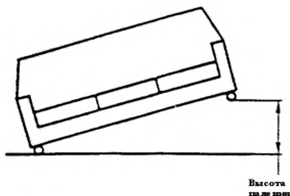
Рисунок 20 — Испытание падением на пол
