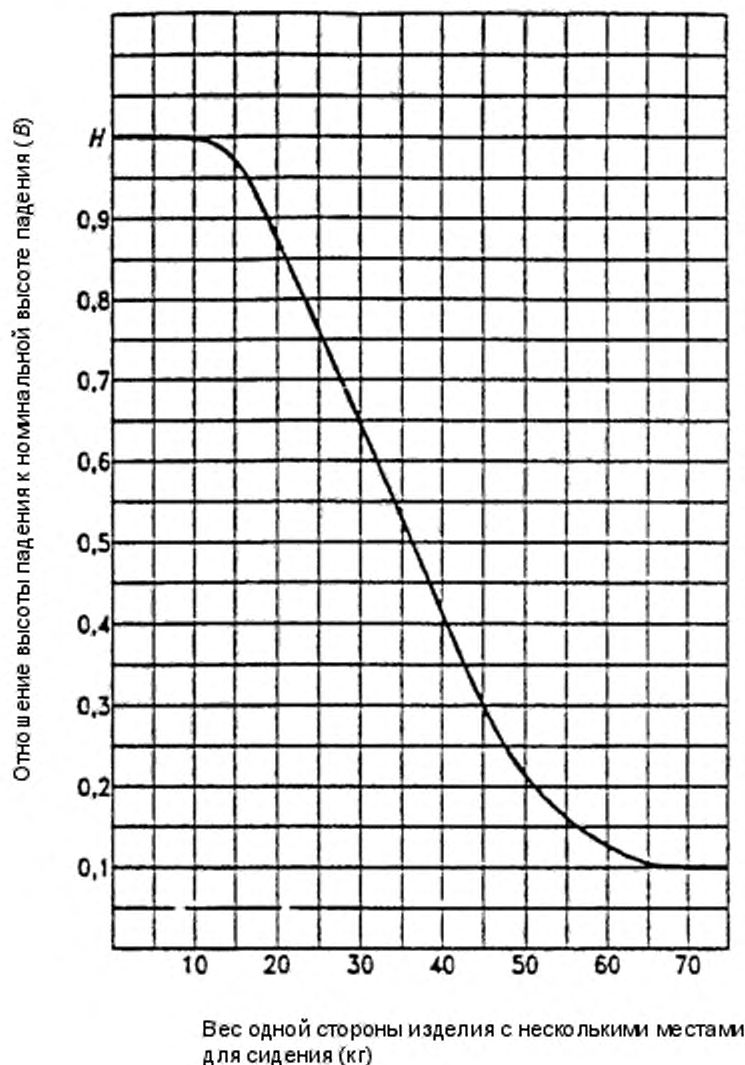
Рисунок 19 – График отношения высоты к весу при испытании падением
