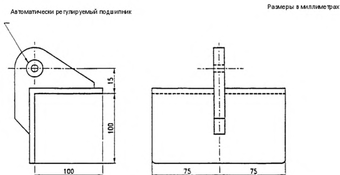
Рисунок 8 — Нагрузочное устройство для испытания на долговечность подлокотника
