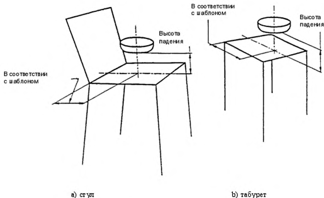
Рисунок 16 — Испытание сиденья на удар
