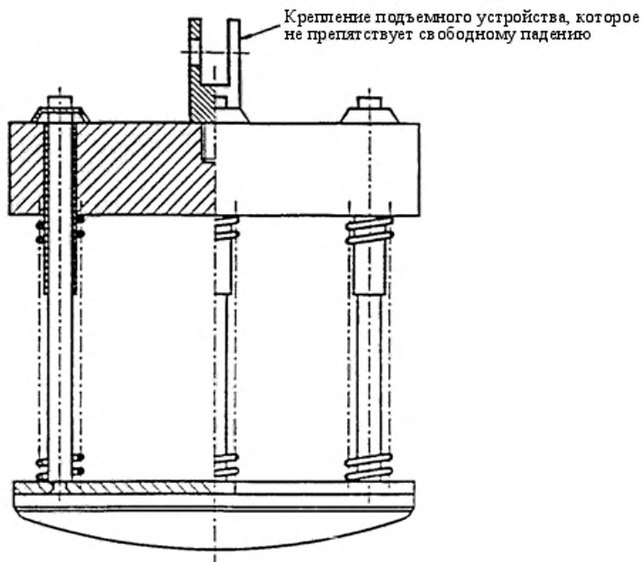
Рисунок 7 — Устройство для испытания на удар
