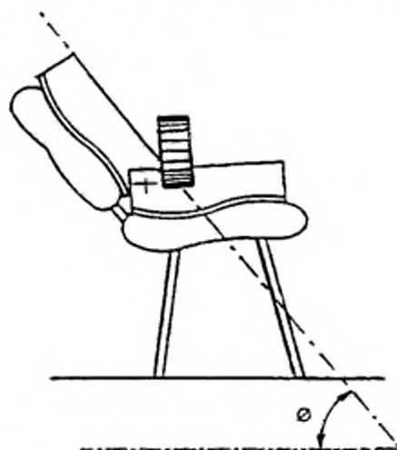
Рисунок 1б — Определение угла наклона спинки ( \Theta )
