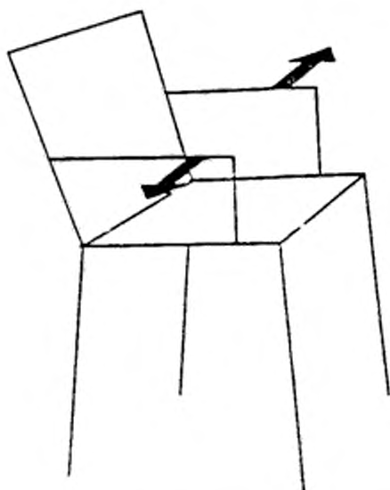
Рисунок 11 — Испытание подлокотников и подголовников под действием статической нагрузки в боковом направлении
