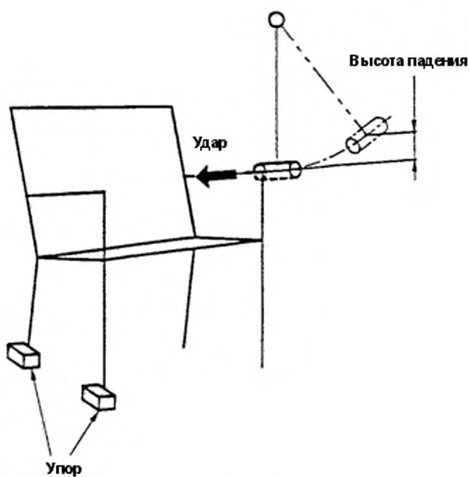
Рисунок 18 — Испытание подлокотника на удар
