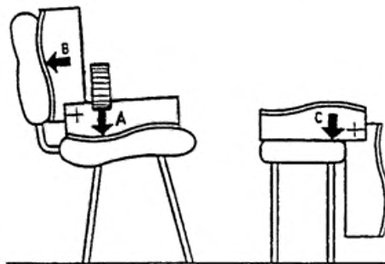
Рисунок 1а — Положение шаблона
