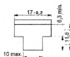
Вид U – показывает максимальные размеры контура защелки
