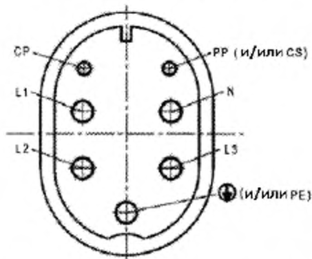
Расположение штырей (вид со стороны штырей)
