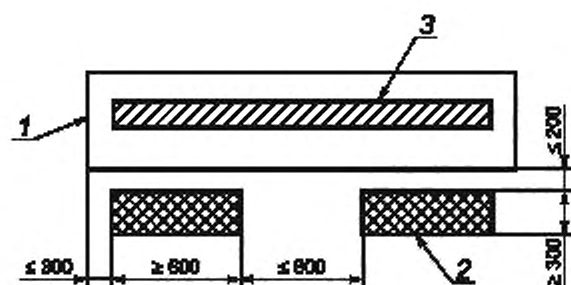
а) Сеялки с бункером высевящего аппарата для загрузки и разравнивания по всей ширине
