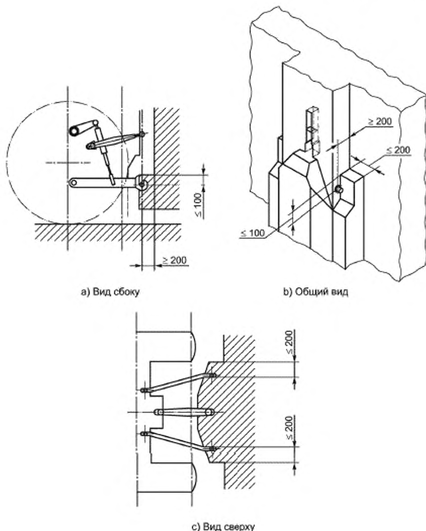
Рисунок 5 — Допустимый просвет
