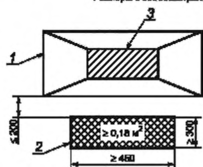
б) Сеялки с бункером высевящего аппарата для центральной загрузки
