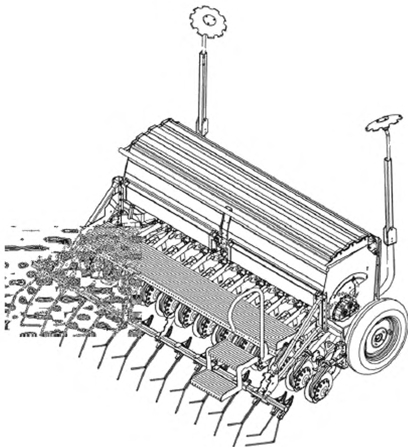
Рисунок В.1 — Механическая сеялка
