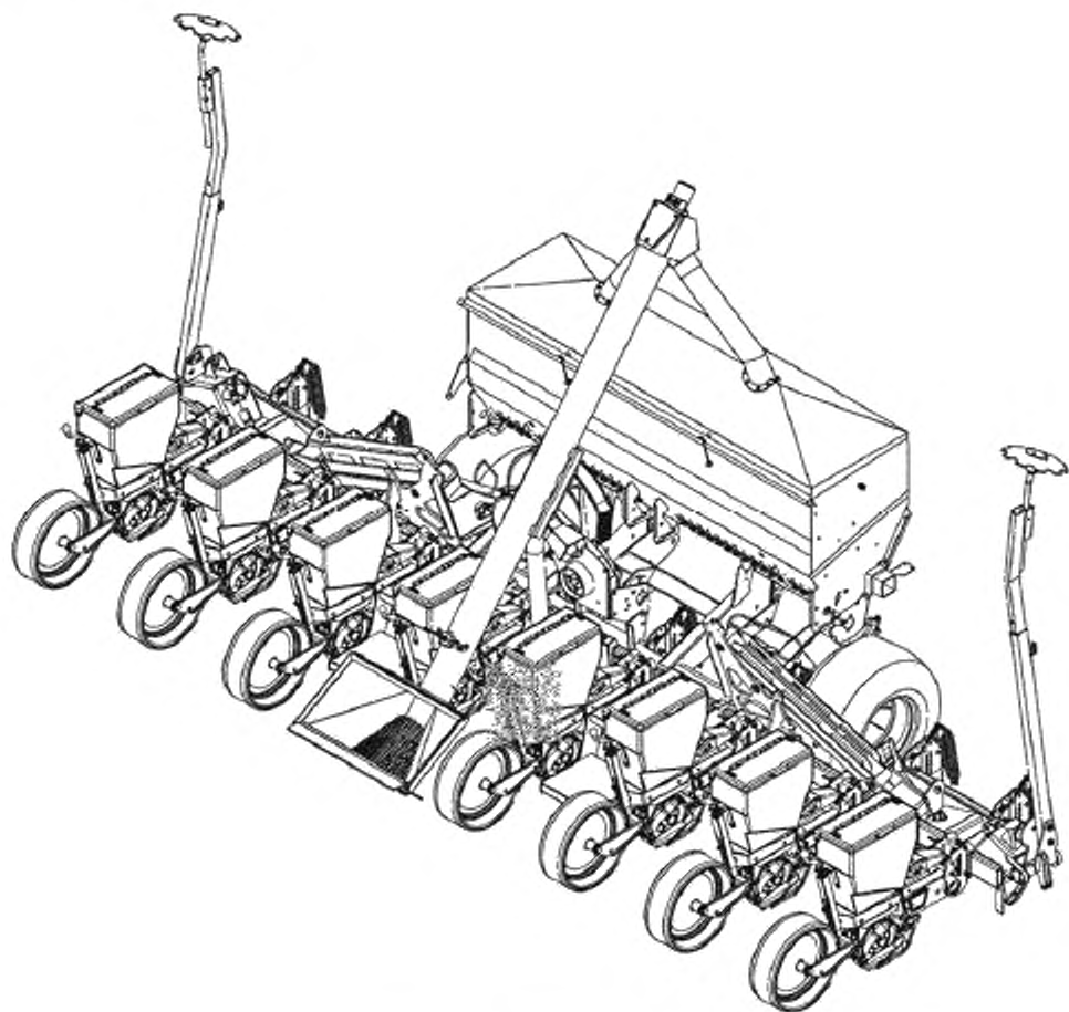
Рисунок В.3 — Сеялка точного высева
