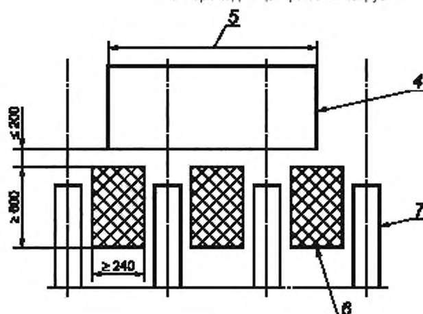
с) Сеялки точного высева с центральным бункером высевящего аппарата
