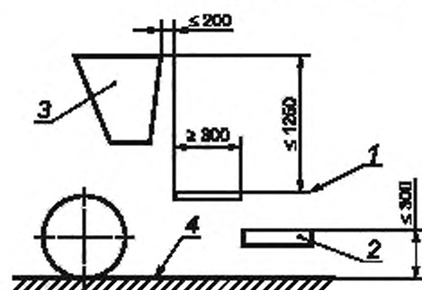
Рисунок 3 — Зона загрузки
