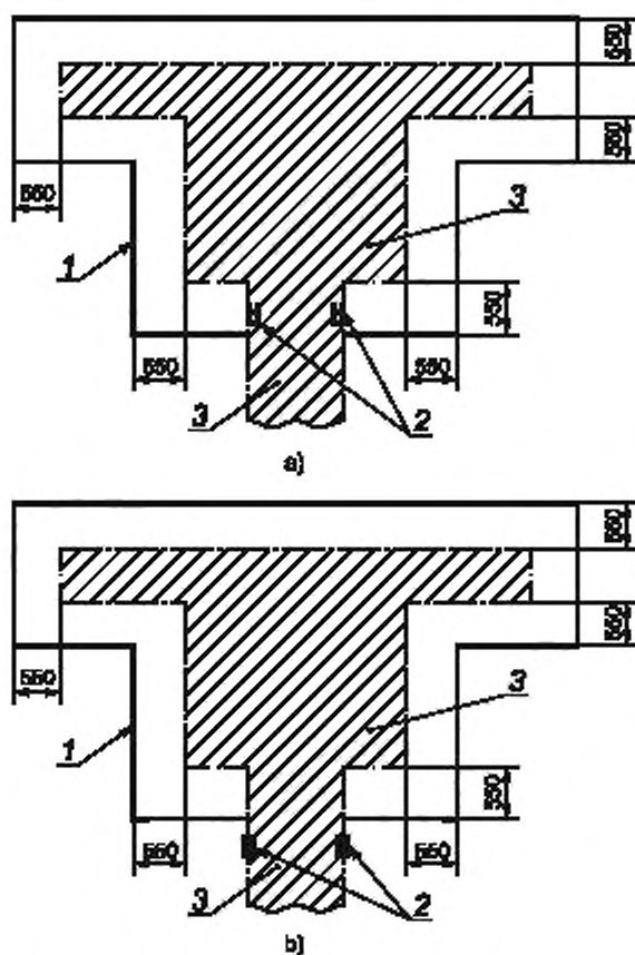
Рисунок 2 — Зона недопустимого расположения ручного управления (для других машин)
