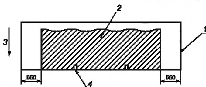
Рисунок 1 — Зона недопустимого расположения ручного управления регулировками (для машин с задней навеской и силовым приводом)
