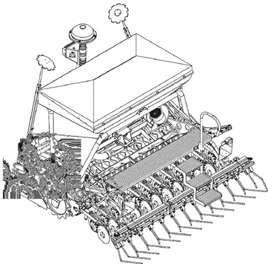
Рисунок В.2 — Пневматическая сеялка
