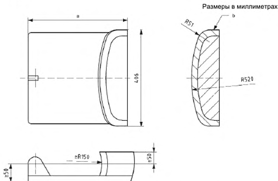
Рисунок 1 – Тяговое устройство
