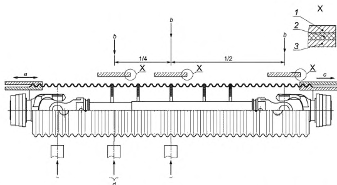
1 — нагрузка; 2 — резина; 3 — деревянный брусок, а — 3,5 Н в течение 60 с (см. D.6); б — при вращении вала с частотой 1000 мин -1 — 500 Н в течение 60 с (см. D.4 и D.5); с — максимальная нагрузка при температуре минус 35 °С (см. D.7); д — удары энергией 98 Дж при температуре минус 35 °С (см. D.8)
