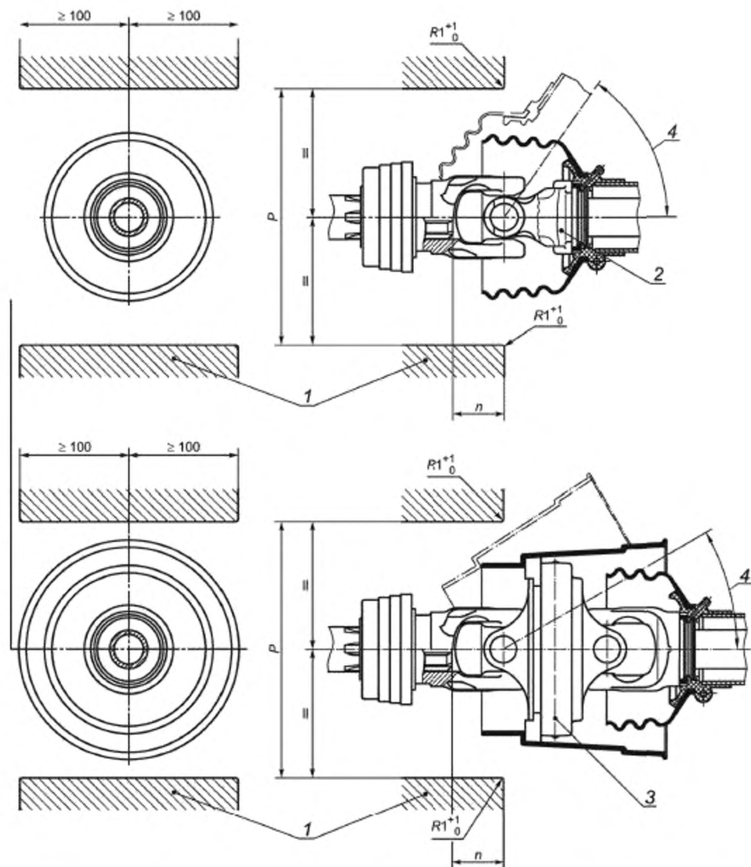
1 — приспособление испытательного стенда; 2 — универсальный карданный шарнир; 3 — широкоугольный универсальный карданный шарнир, 4 — максимальный угол складывания
