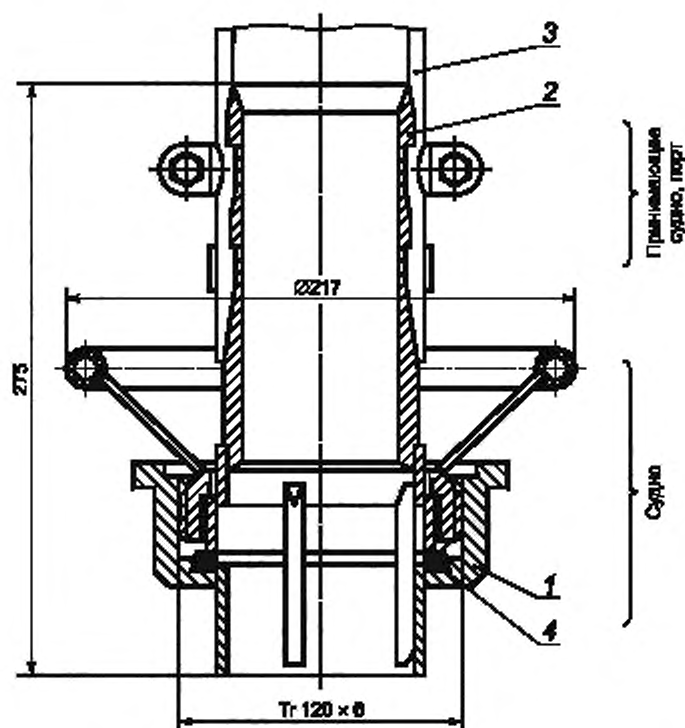
Рисунок 3 — Быстроразъемное соединение DN 80 для нефтеводяной смеси
