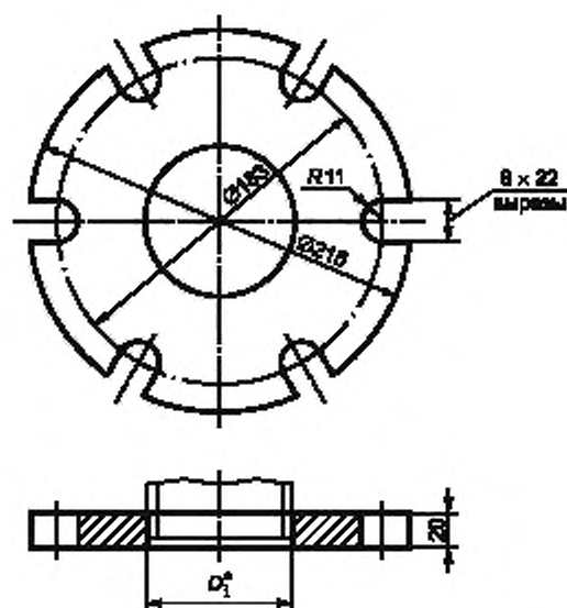
Рисунок 1 — Фланец соединения для нефтеводяной смеси
