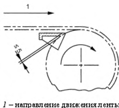
Рисунок 9 б) – Конструкция из листового металла
