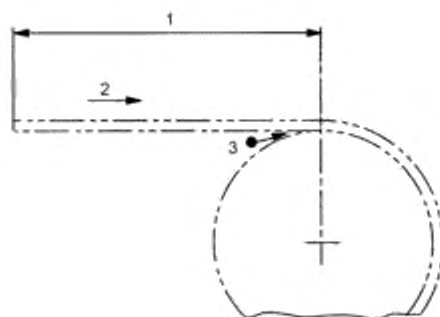
Рисунок 2 – Типовое защитное ограждение вокруг вертикального натяжного устройства
